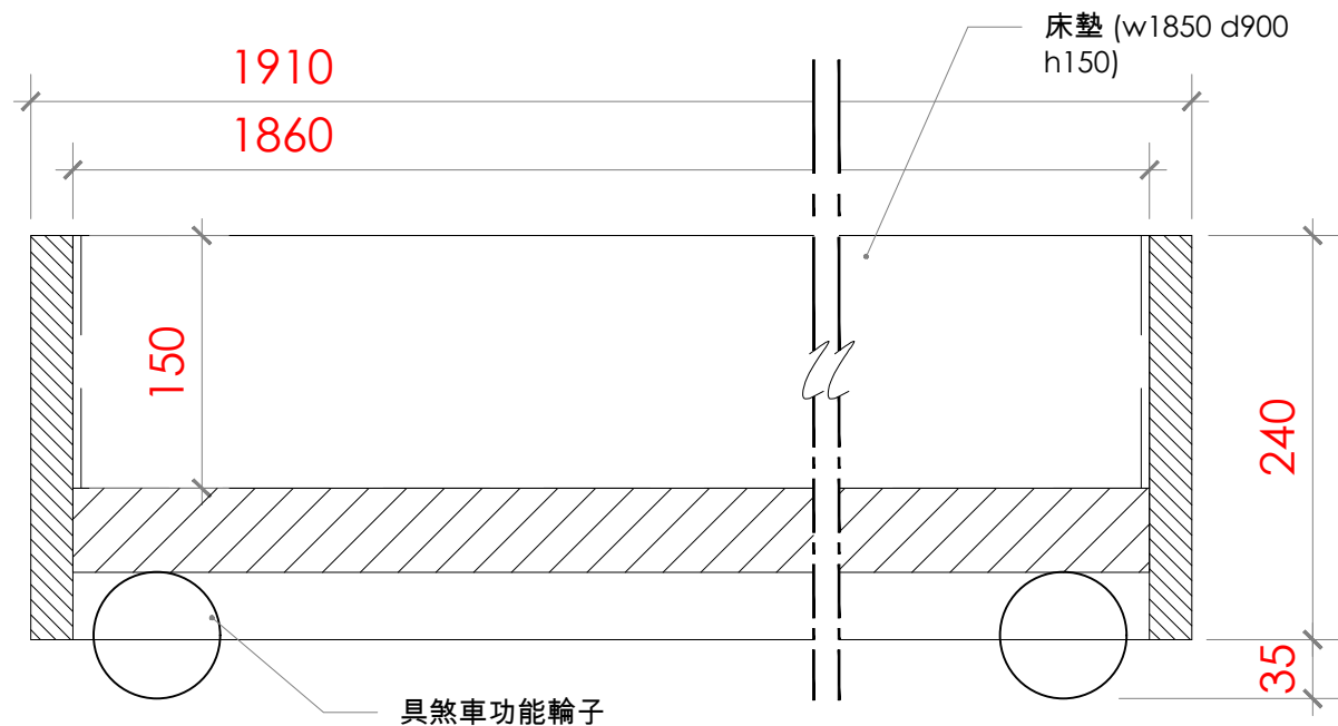
1 DE-08 大樣圖 Scale A3=1:10
