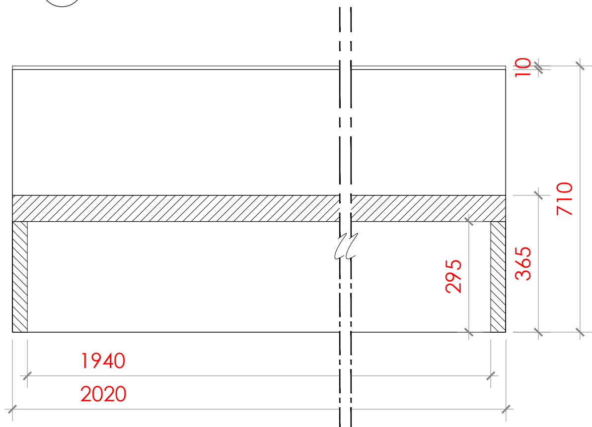
1 DE-07 大樣圖 Scale A3=1:10
