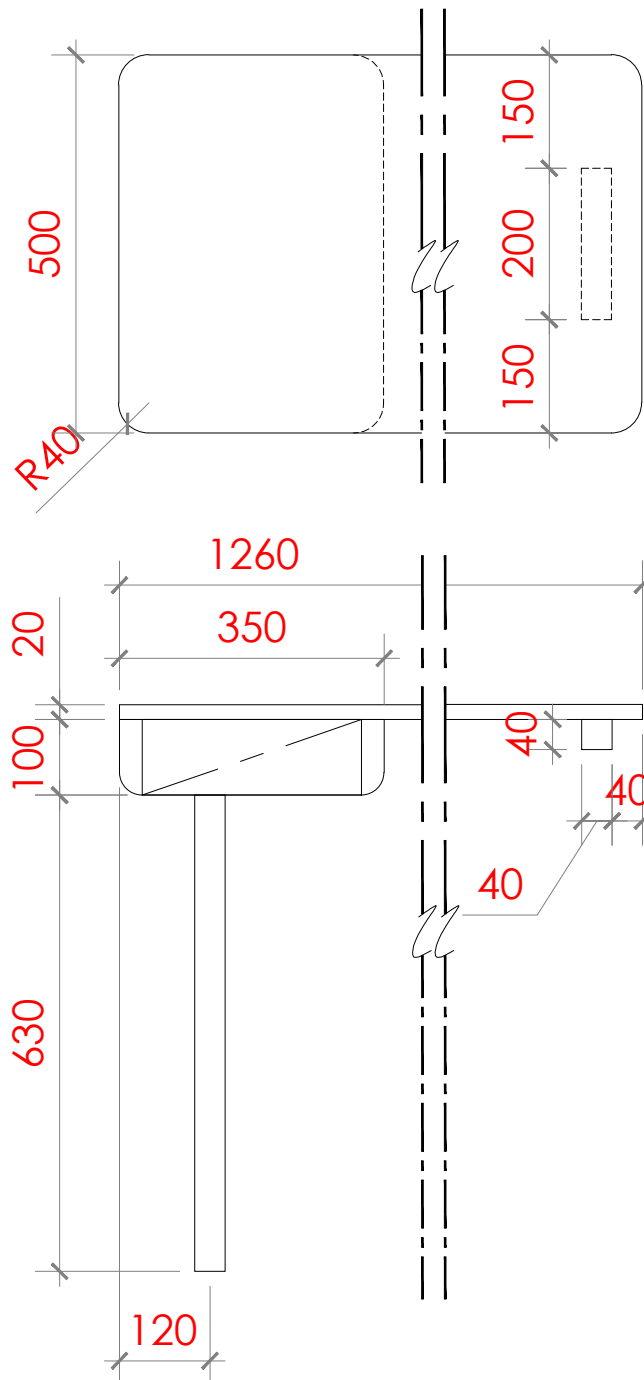
2 DE-07 大樣圖 Scale A3=1:10
