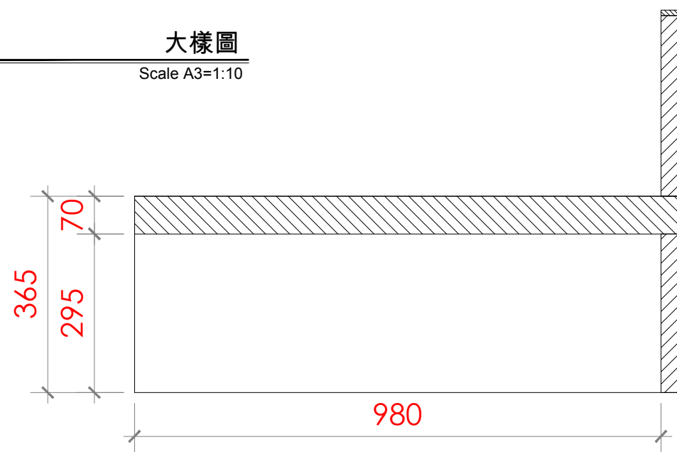
b DE-07 大樣圖 Scale A3=1:10
