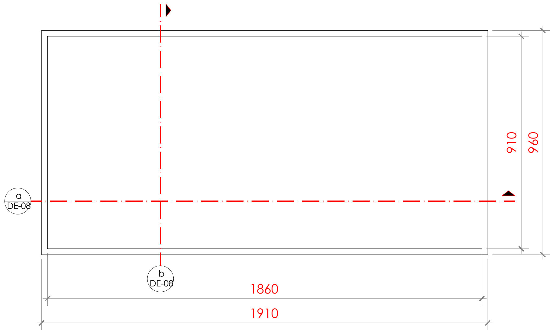
1 DE-08 大樣圖 Scale A3=1:10
