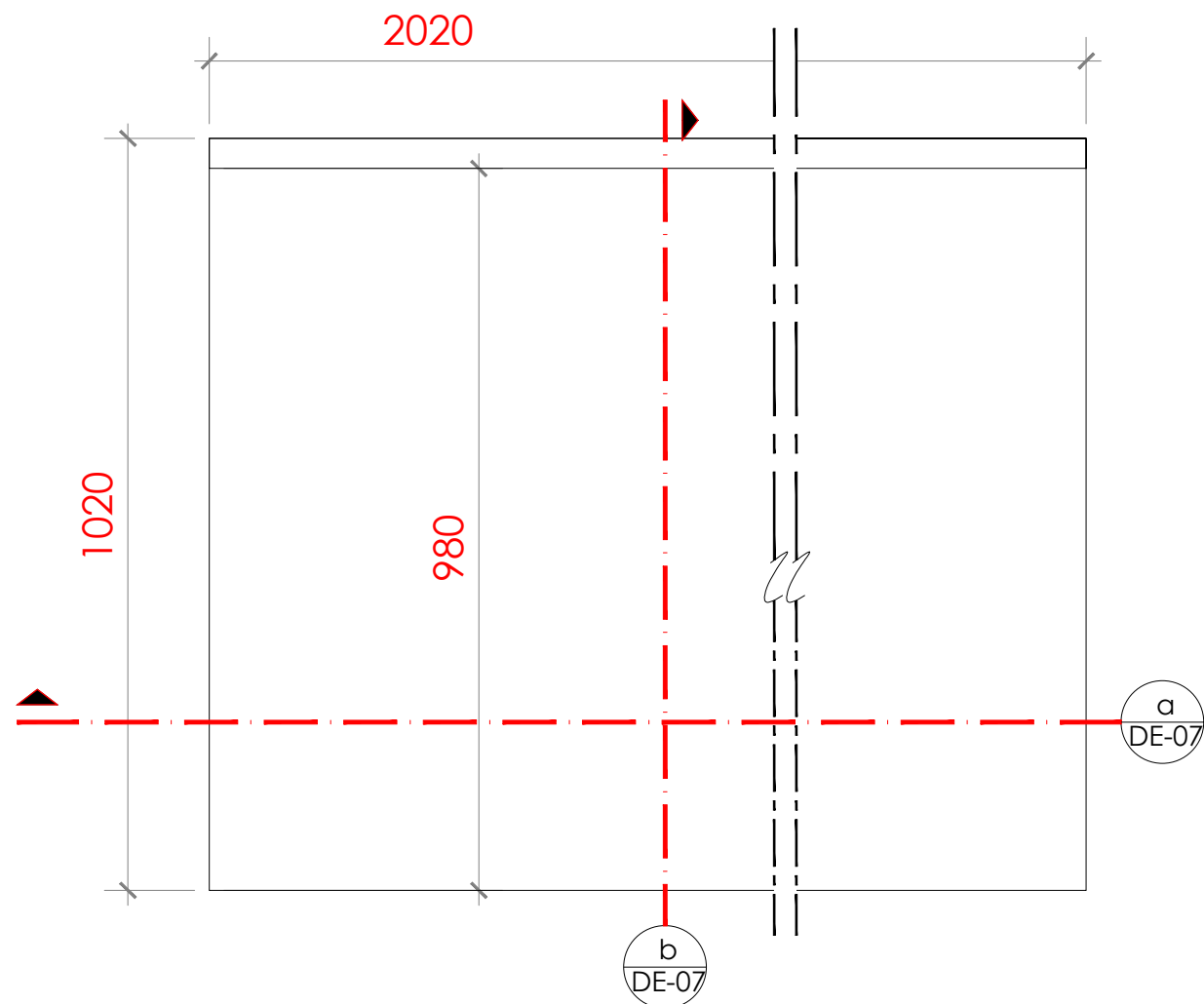
1 DE-07 大樣圖 Scale A3=1:10
