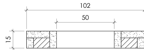
b DETAIL S 1:2
