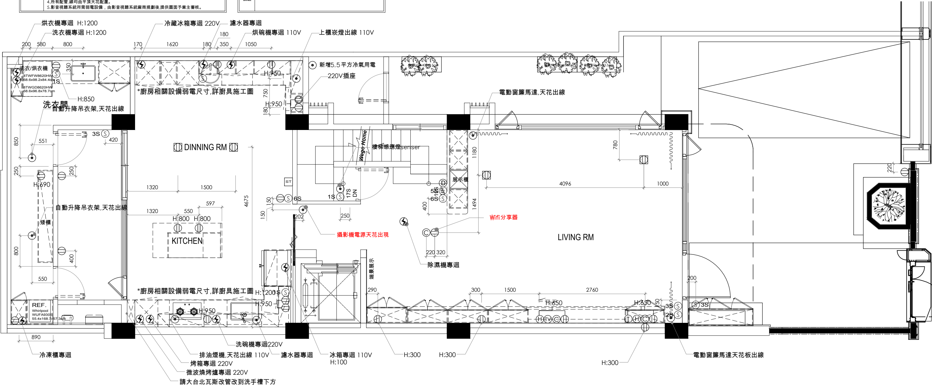
一層平面圖
