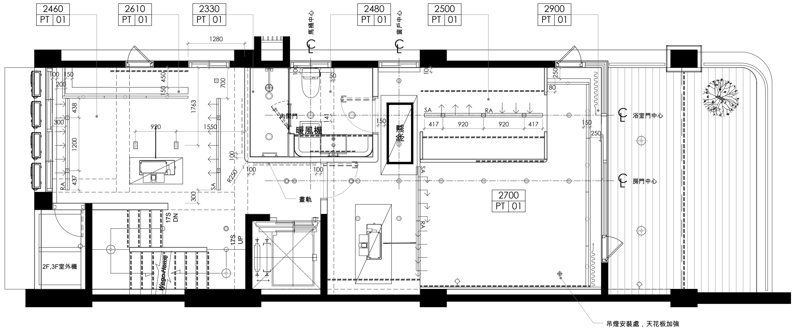
三層平面圖
