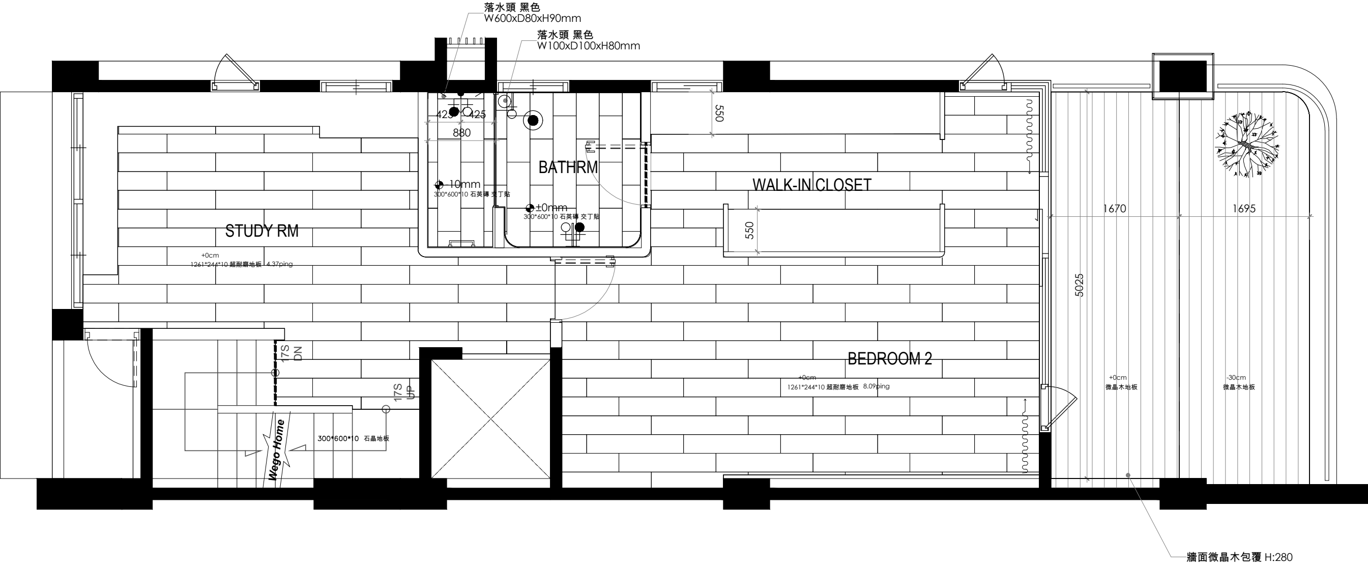
三層平面圖
