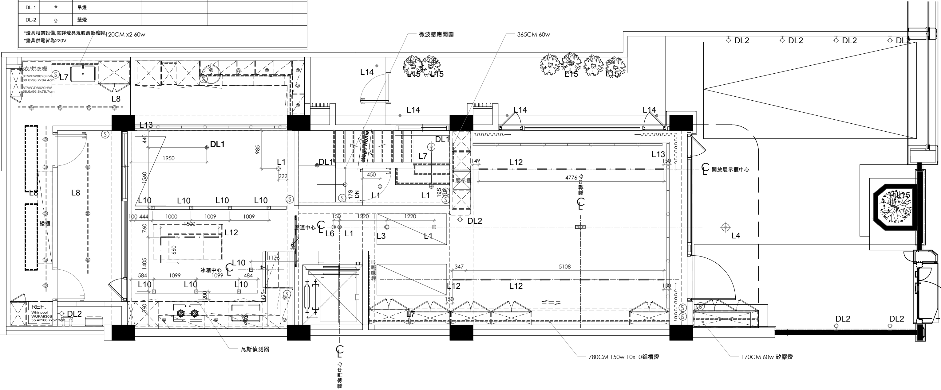
一層平面圖
