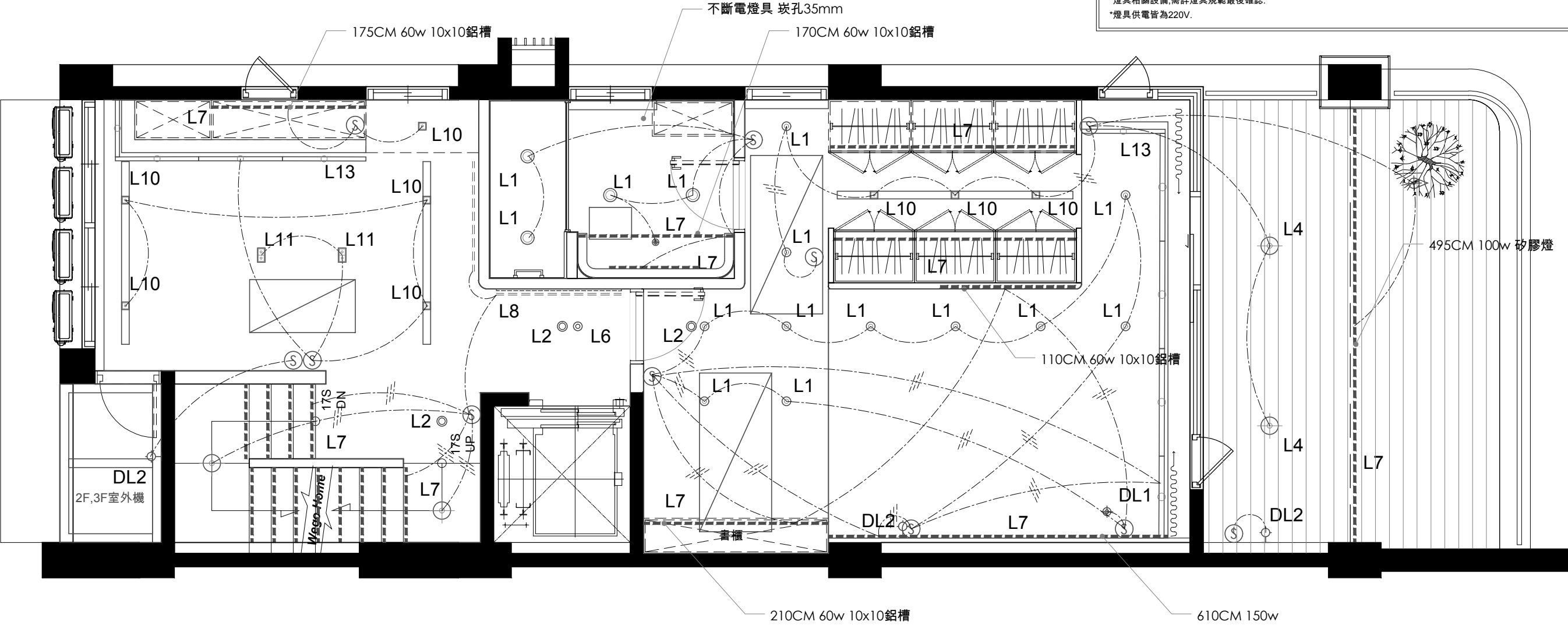
三層平面圖
