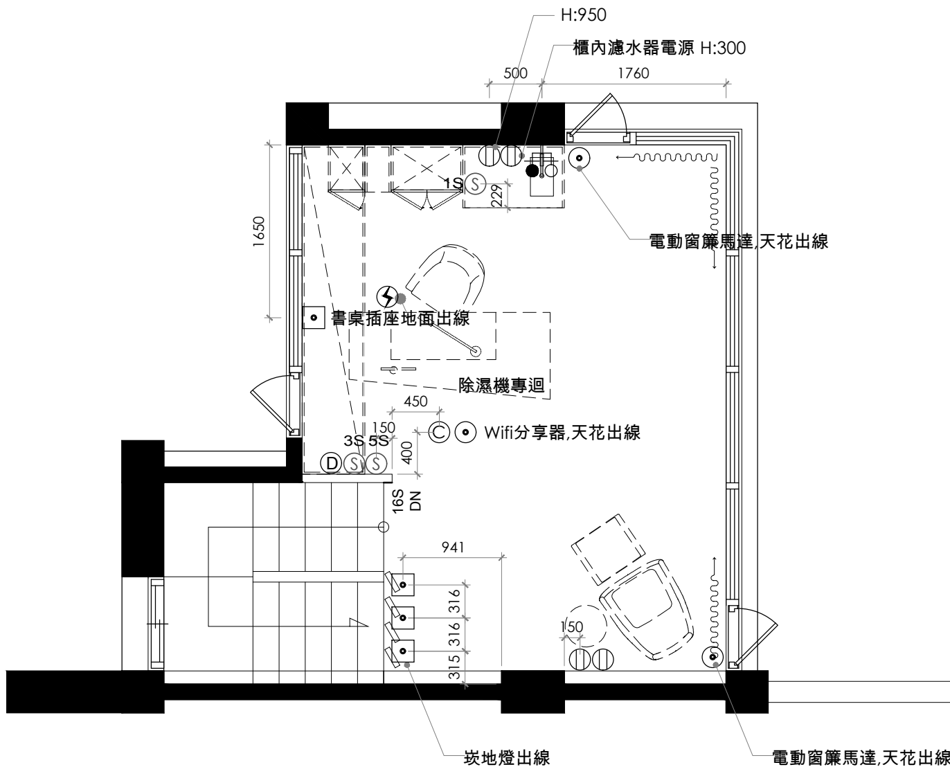
突二層平面圖
