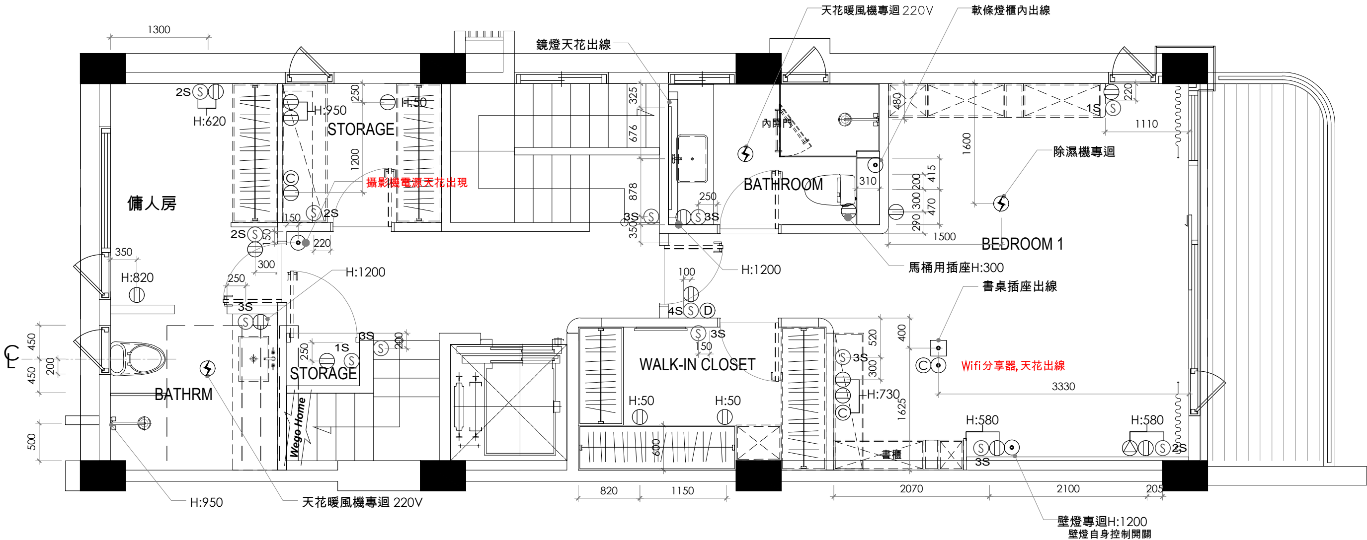
二層平面圖
