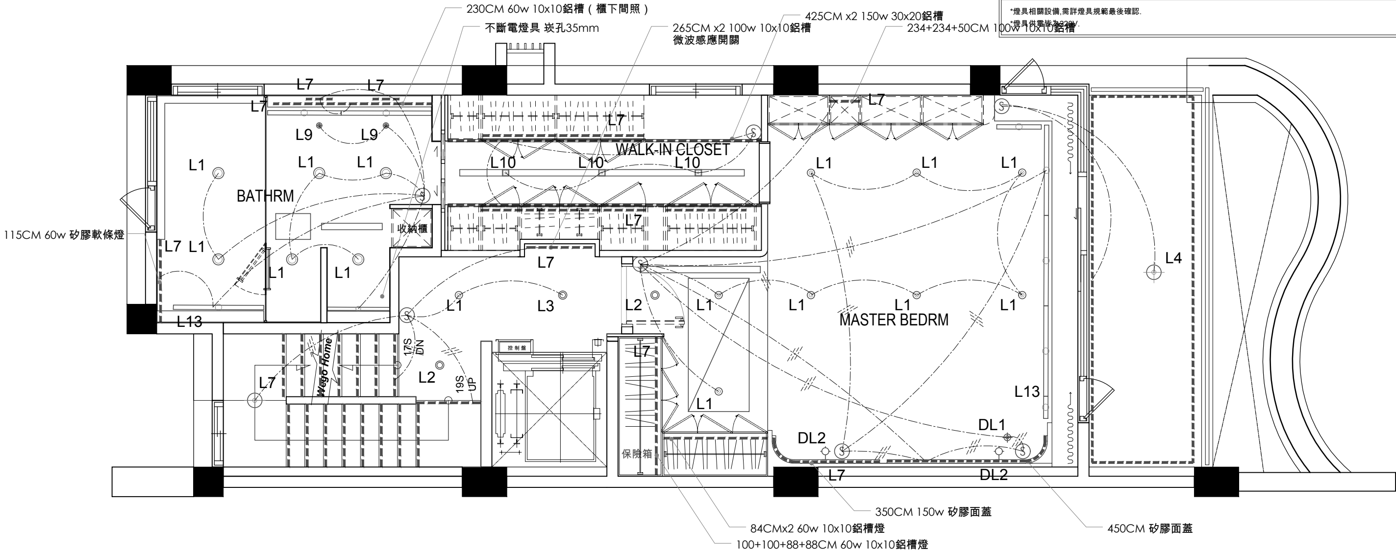
四層平面圖
