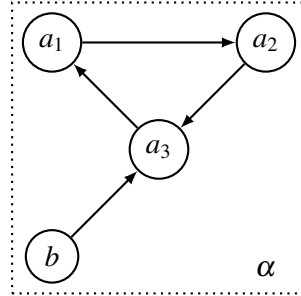
Fig. 9. An AAF.
