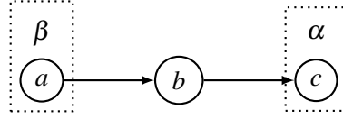
Fig. 11. An AAF
