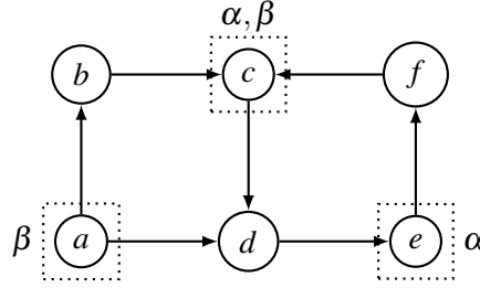
Fig. 16. An AAF
