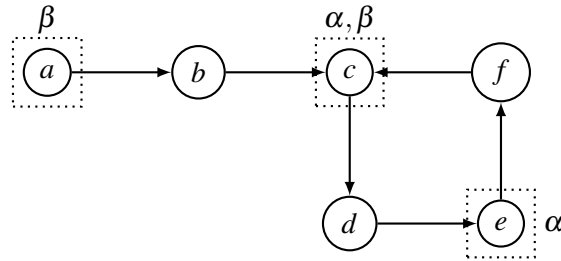
Fig. 15. An AAF
