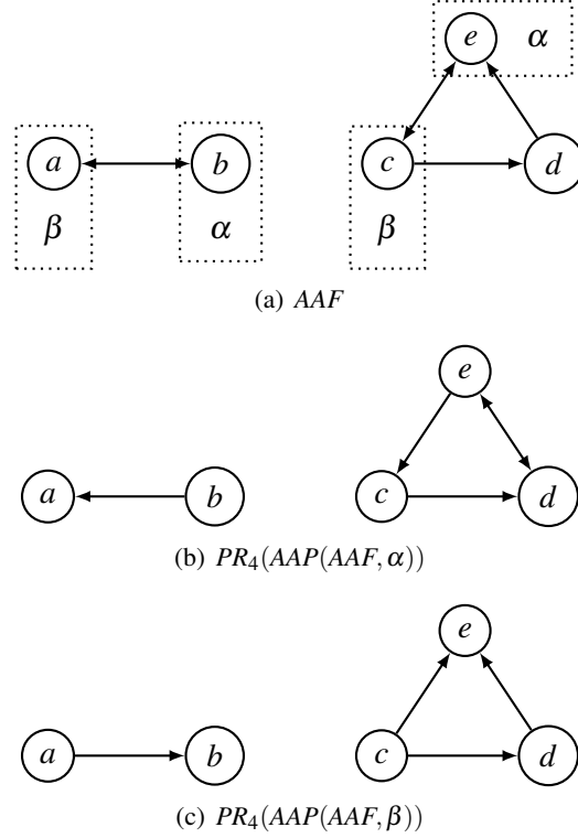
Fig. 13. A counterexample for Prop. 8.
