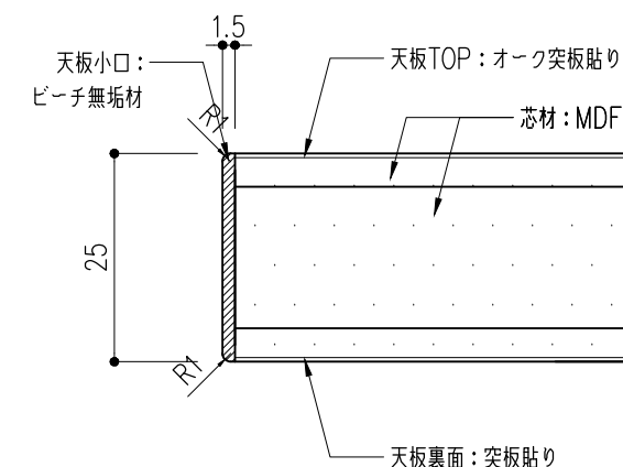
【天板TOP SQ】 S=1:1
