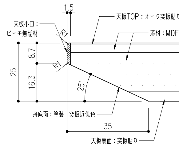
【天板TOP TA】 S=1:1
