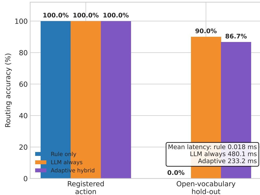
A. LLM generalization benefit
