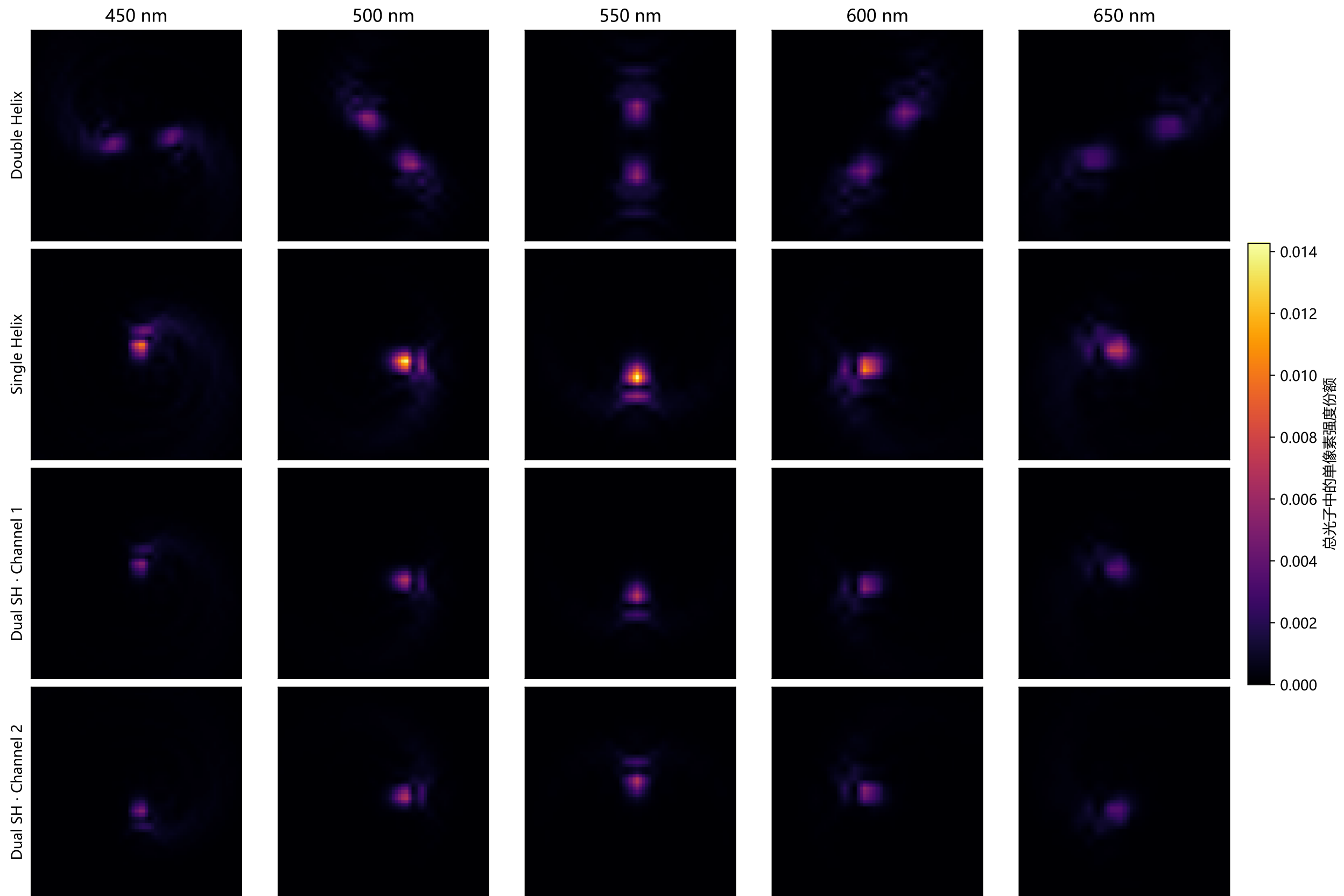
Figure 2 五个代表波长下的 PSF 强度分布 (统一总光子标度)
