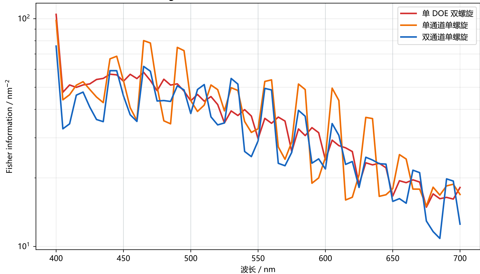
Figure 4 相同总光子预算下的波长 Fisher 信息
