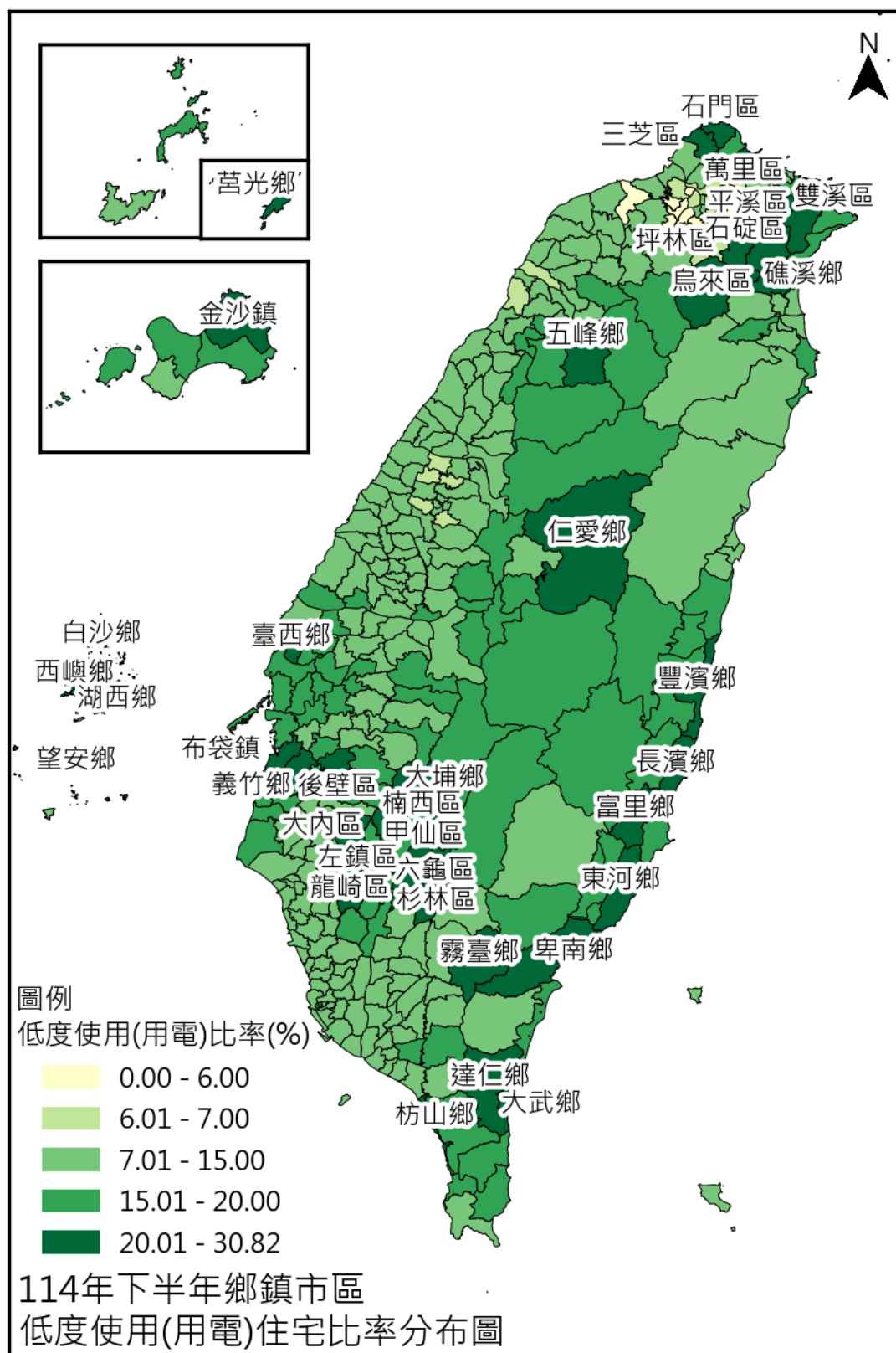
圖 6 114 年下半年鄉鎮市區低度使用(用電)住宅比率分布圖
