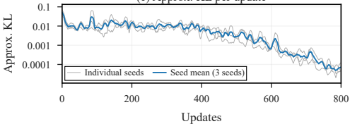
(c) Approx. KL per update
