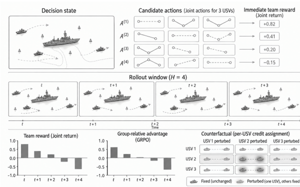
Figure 8: 그룹 상대 최적화의 한 갱신(도식은 G = 4, H = 4 )
