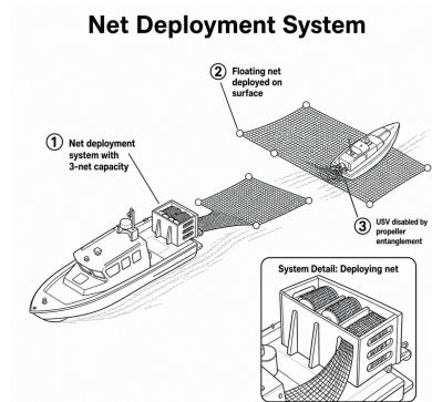
Figure 3: 후미 투하식 부유 그물의 포획 개념
