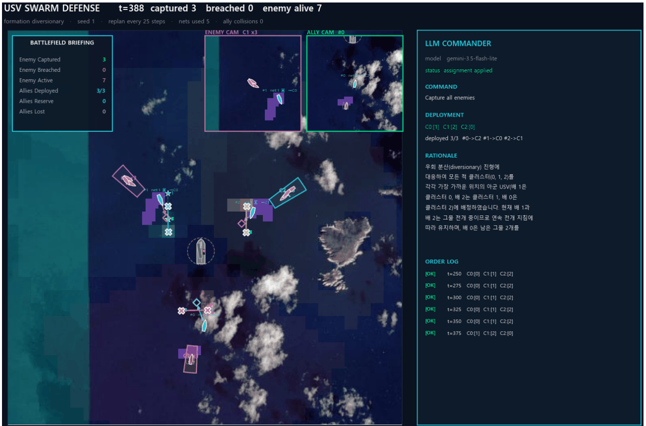
Figure 17: 실행 화면(양동 포메이션, Gemini 지휘관, 재계획 주기 25 step). 왼쪽은 위성 영상 위에 육지 마스크·그물벽·요격 회랑을 겹친 전장과 적/아군 확대 창이고, 오른쪽은 지휘관이 낸 배정과 그 근거이다. 상단 표시에서 이 시점의 전과(포획 3, 돌파 0, 아군 총돌 0)를 확인할 수 있다.
