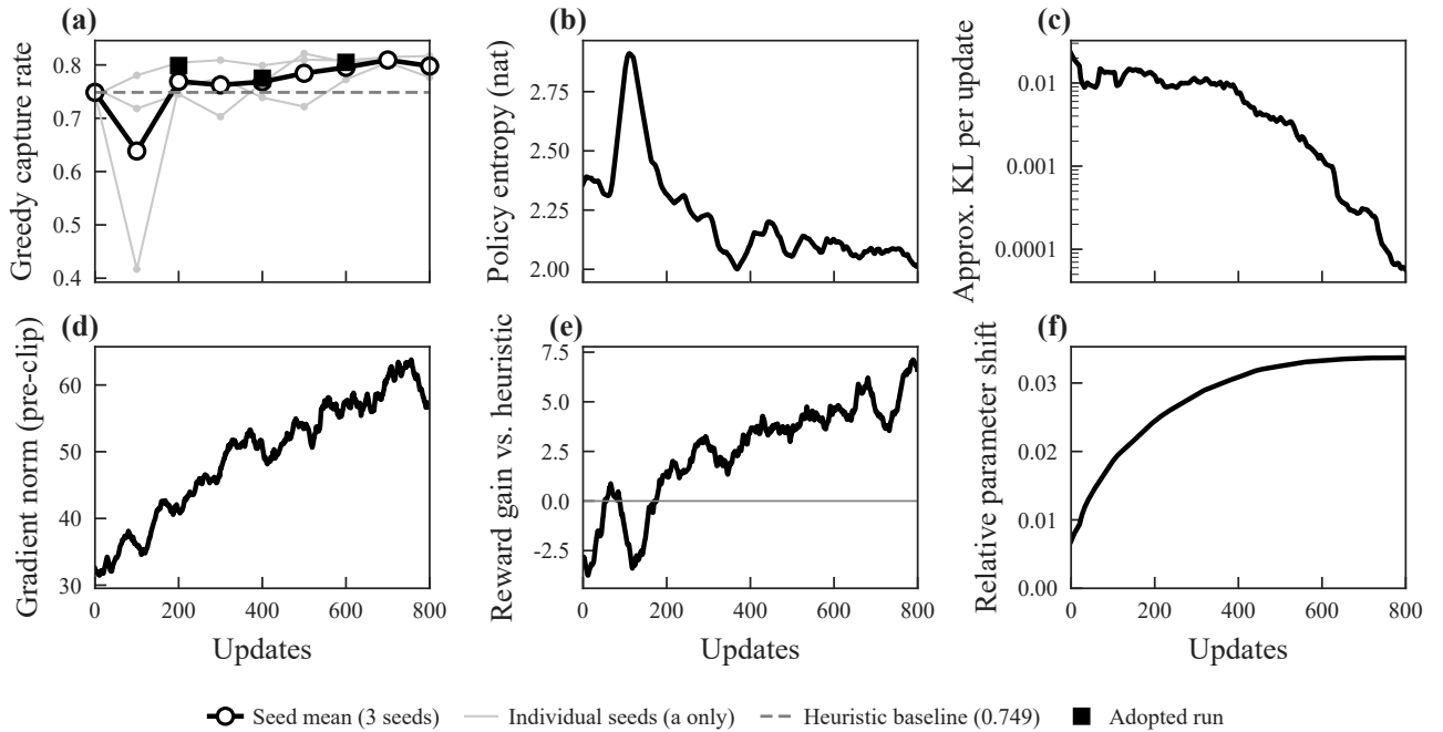
Figure 15: 수렴 진단 — 채택 런과 같은 설정을 시드 3개로 다시 돌린 학습 동역학. 검정 굵은 선은 시드 평균(40 업데이트 이동평균)이며, 시드별 꺾은선은 (a)에만 연회색으로 두었다. (a) 100 업데이트마다의 greedy 포획률(연회색은 시드별, 빈 원은 평균, 채운 사각형은 채택 런의 평가점, 파선은 같은 프로토콜로 랜 휴리스틱 기준선 0.749). (b) 1단계 픽셀 분포의 엔트로피. 유효 픽셀 중앙값 273개의 균일분포 상한은 \ln 273 \approx 5.6 nat로 축 밖에 있다. (c) 갱신 전후 정책의 근사 KL 발산(같은 관측·같은 표본 후보, 로그축). (d) 클리핑 전 그래디언트 노름 — 800 업데이트 내내 클립 한계 1.0의 수십 배라 수렴 지표가 아니다. (e) 표본 후보 보상에서 휴리스틱 후보 보상을 뺀 값. 0을 넘으면 정책의 표본이 휴리스틱을 앞선다. (f) 행동복제 초기점으로부터의 상대 파라미터 이동 거리.
