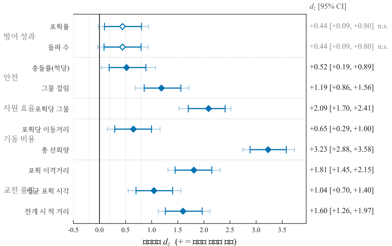
Figure 19: 제안(11m_unet@Gemini) 대 기준선(heur_heur)의 전 지표 효과크기. 마름모가 점추정이고, 굵은 선이 95% 신뢰 구간, 그 바깥의 얇은 선이 지표 10개에 대한 Bonferroni 보정 구간(99.5%)이다. 속이 찬 표식은 보정 구간까지 0을 배제한 지표이며, 속이 빈 둘(포획률·돌파 수)은 보정을 견디지 못해 n.s.로 적었다 — Table 9의 단검 표시와 같은 판정이다. 부호는 개선 방향이 항상 양수가 되도록 통일하였다(낮을수록 좋은 지표는 뒤집었다). d_z 의 구간은 평균차의 BCa 신뢰구간을 sd(d) 로 나눈 것이므로, 이 그림이 0을 배제하는 것과 Table 9의 평균차 구간이 0을 배제하는 것은 같은 사건이다. 포획률의 효과크기가 10개 지표 중 최하위권이라는 점이 이 그림의 요지이다.
