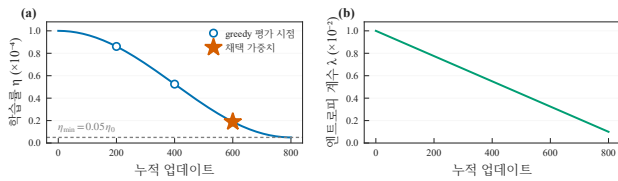
Figure 16: 학습 코드가 실제로 쓴 스케줄. (a) 식 (42)의 단일 주기 코사인 학습률. 원 표식은 200 업데이트마다의 greedy 평가 시점, 별표는 채택 가중치(600 업데이트, \eta_t \approx 1.9 \times 10^{-5} ), 회색 파선은 \eta_{\min} 이다. (b) 엔트로피 계수 \lambda_H(t) 의 선형 감쇠 (0.01 \rightarrow 0.001).
