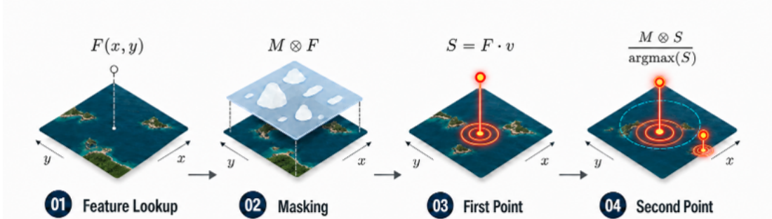
Figure 10: 점수맵 위 픽셀 지목의 네 단계. ① 복호기가 낸 픽셀별 특징 F(x, y) . ② 유효 마스크 M 을 곱해 놓을 수 없는 칸을 차단한다 (§4.4.3). ③ 질의 \mathbf{v} 와의 내적으로 점수맵 S = F \cdot \mathbf{v} 를 얻고 최대 칸을 첫 점으로 고른다. ④ 첫 점의 특징을 질의에 더해( \mathbf{q} \leftarrow \mathbf{q} + \mathbf{f}_0 ) 같은 절차로 두 번째 점을 고르되, 첫 점과의 간격 상·하한(파선 원)을 마스크에 추가한다. 두 점을 잇는 선분이 그물벽이다.
