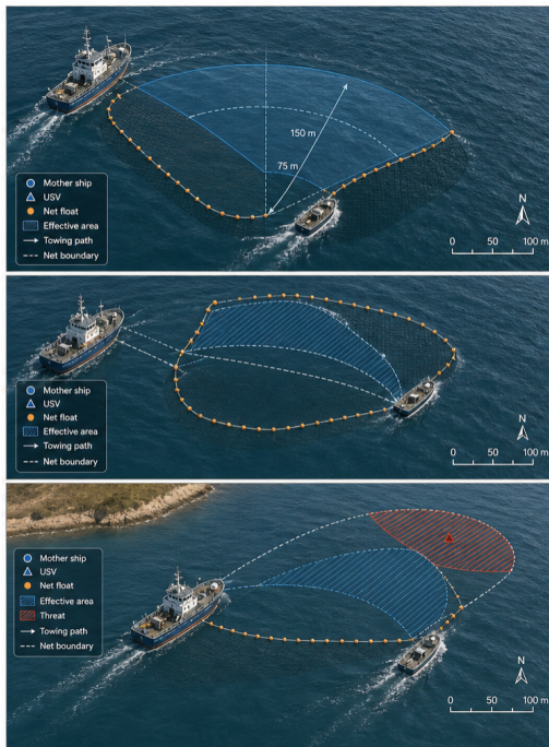
Figure 23: 실제 그물 전개가 갖는 형상(참고). 두 척이 그물을 예인하면 벽이 아니라 곡선으로 펼쳐진 면적이 만들어지고, 그 면적이 위협 방향과 얼마나 겹치는지가 차단 성능을 좌우한다. 본 연구의 모형은 이를 단순화하여, 방어진 한 척이 두 좌표를 잇는 직선 그물벽을 치고 그 선분에 적선이 닿으면 포획되는 것으로 처리한다. 전개 곡률, 예인 편대, 면적의 시간 변화는 반영하지 않는다. 그림의 치수 또한 개념 전달을 위한 것으로 본 연구의 설정(최대 450 m)과 다르다.
