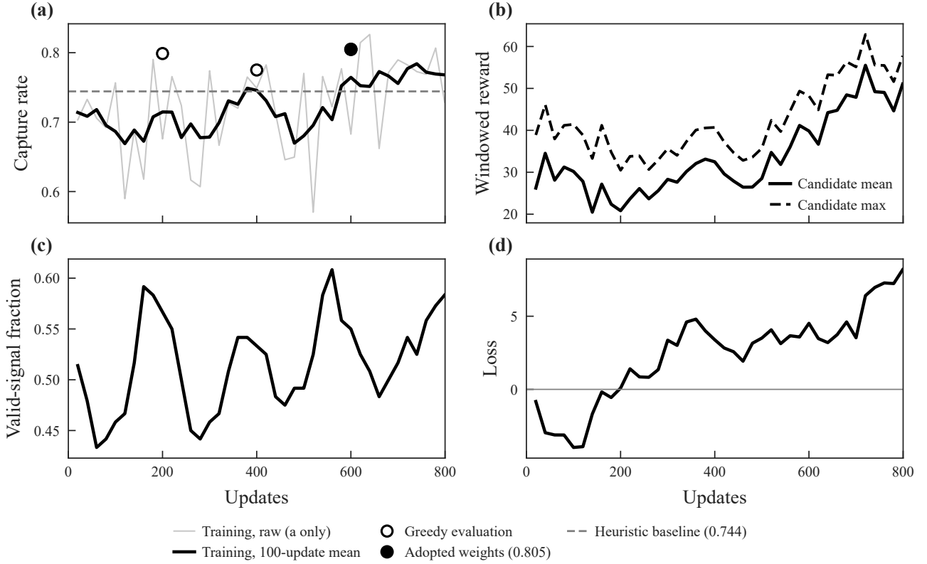
Figure 14: GRPO 학습 경과( 50^2 격자, 후보 G = 8 , 후보 평가 구간 180 step, 실해역 6곳 로테이션(Fig. 12), 800 업데이트). 검정 굵은 선은 20 업데이트마다 기록한 원자료의 100 업데이트 이동평균이며, (a)에만 원자료를 연회색 가는 선으로 함께 두었다. (a) 포획률(Capture rate). 원 표식은 200 업데이트마다의 greedy 평가, 파선은 휴리스틱 기준선 0.744이다. 채운 원(600 업데이트, 0.805) 이 본 논문이 평가하는 가중치이다. (b) 후보 평균 보상(실선)과 후보 최대 보상(파선) — 둘의 간격이 그룹 내 변별력이다. (c) 후보 간 분산이 0이 아닌 월드의 비율(Valid-signal fraction; 학습 신호가 실제로 생긴 비율). (d) 손실(정책경사 + 엔트로피). 부호와 크기 자체는 수렴 지표가 아니다.
