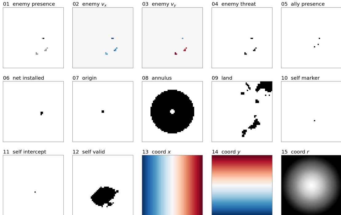
Figure 4: 래스터화된 15채널 관측의 한 장면(파상 포메이션, 통영 매물도 북측, t = 320 , 학습·평가와 같은 50 \times 50 격자). 01–09는 전역 채널(적 밀도, 적 진행 x \cdot y , 적 위협도, 아군 위치, 설치된 그물, 원점, 요격 환형, 육지), 10–12는 방어정 0의 채널(자기 위치, 배정 요격점, 유효 영역), 13–15는 좌표 채널( x, y, r )이며 모두 같은 격자에 정렬된다. 부호 없는 채널은 값이 클수록 검게, 부호 있는 채널( v_x, v_y , 좌표 x \cdot y )은 음을 파랑·양을 빨강으로 그렸다. 채널의 정의와 값 범위는 Table 4에 있다.
