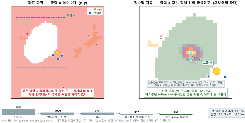
Figure 9: 왜 좌표 회귀가 아니라 점수맵 위 픽셀 지목인가(학습된 체크포인트의 실제 출력). 왼쪽: 연속 좌표를 회귀하는 출력에는 “놓을 수 없는 곳”을 표현할 자리가 없다 — 이 장면에서 붉은 영역이 격자의 88.0%다. 오른쪽: 같은 장면을 후보 영역으로 확대한 점수 분포와 선택된 두 픽셀, 그리고 그 둘을 잇는 그물벽이다. 마스킹된 softmax 아래에서 부적합한 칸은 확률이 0이라 애초에 선택되지 않는다. 아래 막대 는 제약이 순차 적용되며 후보가 줄어드는 과정이다 (2500 → 1000 → 979 → 387 → 299, 12.0%). 전 결정 평균 후보는 10.5%였다.
