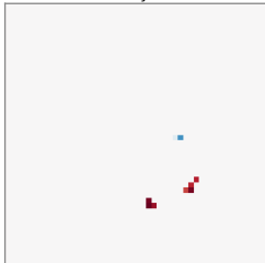
03 enemy v_y
