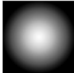
15 coord r
