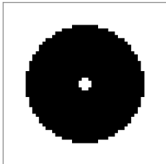
08 annulus
