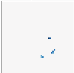
02 enemy v_x
