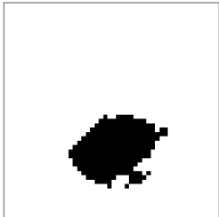
12 self valid
