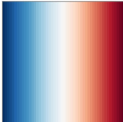
13 coord x
