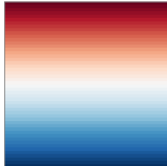
14 coord y
