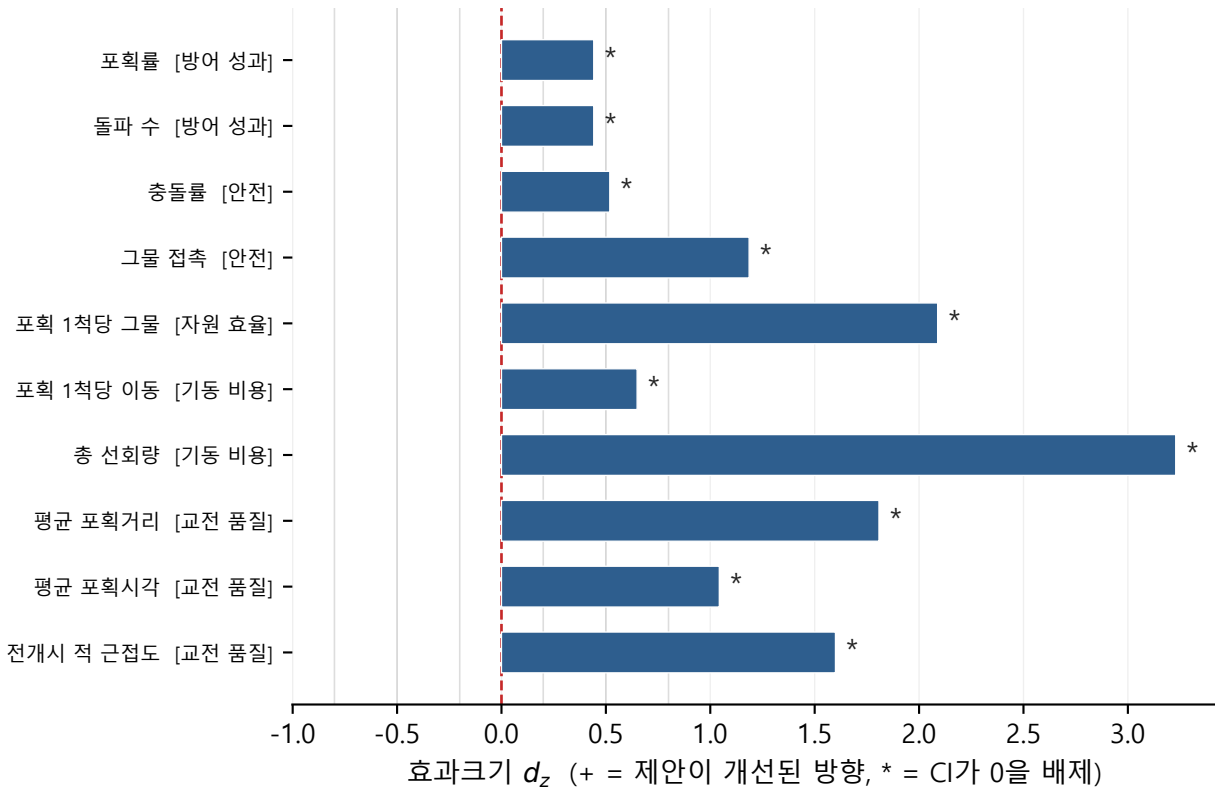
LLM +U-Net (gemini-3.5-flash-lite) vs 휴리스틱 +휴리스틱 — 전 지표 효과크기
