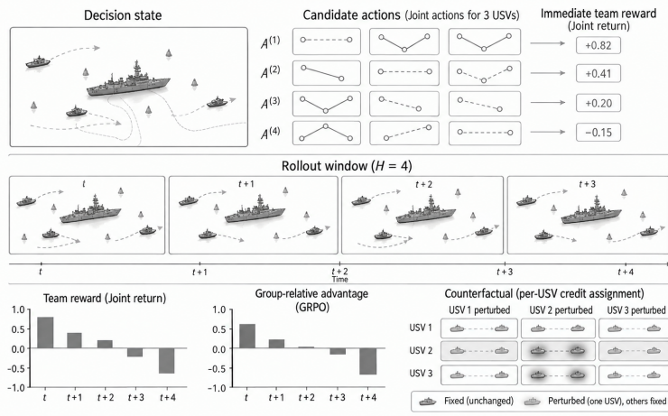
Figure 12: 가치망 없는 그룹 상대 최적화의 한 갱신 — 후보 표집(위), 몰아웃 창 평가(가운데), 상대 비교와 반사실적 크레딧(아래)
