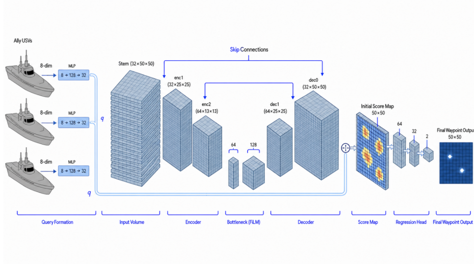
Figure 9: 점수맵 정책의 구조 — 방어정 상태 질의와 U-Net 특징맵의 내적으로 얻는 점수맵과 부화소 오프셋
