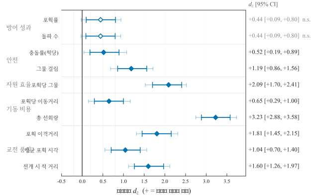
Figure 16: 제언(11m_unet@Gemini) 대 기준선(heur_heur)의 전 지표 효과크기. 마름모가 점추정이고, 굵은 선이 95 % 신뢰구간 , 그 바깥의 얇은 선이 10개에 대한 Bonferroni 보정 구간(99.5 %) 이다. 속이 찬 표식은 보정 구간까지 0을 배제한 지표 이며, 속이 빈 둘(포획률·돌파 수)은 보정을 건디지 못해 n.s.로 적었다 — Table 9의 단검 표시와 같은 판정이다. 부호는 개선 방향이 항상 양수가 되도록 통일하였다(낮을수록 좋은 지표는 뒤집었다). d_z 의 구간은 평균차의 BCa 신뢰구간을 sd(d) 로 나눈 것이므로, 이 그림이 0을 배제하는 것과 Table 9의 평균차 구간이 0을 배제하는 것은 같은 사건이다. 포획률의 효과크기가 10개 지표 중 최하위권 이라는 점이 이 그림의 요지이다.
