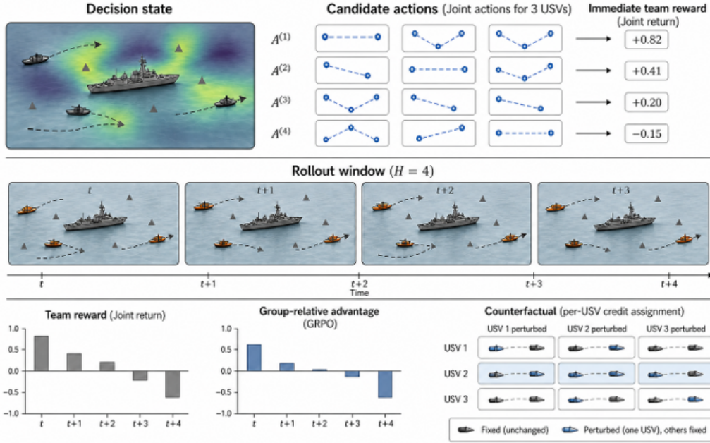
Figure 10: 가치망 없는 다중 방어정 그룹 상대 최적화의 한 갱신. 위: 한 결정 상태에서 G 개의 결합 행동 후보를 표집하고, 각 후보를 시뮬레이터에서 공통 구간만큼 실제로 진행시켜 팀 보상을 얻는다. 가운데: 후보 평가에 쓰이는 롤아웃 창. 아래 왼쪽·가운데: 팀 보상을 후보 간 상대 비교로 이득으로 바꾼다 (식 (26)). 아래 오른쪽: 반사실적 크레딧 — 한 척의 행동만 바꾸고 나머지는 고정된 채 시뮬레이터를 다시 진행시켜, 그 차이를 그 배의 몫으로 돌린다 (§4.5; 구현된 변형이며 채택 런은 팀 이득 손실을 썼다). 그림은 기전 전달을 위해 후보 수와 창을 G = 4 , H = 4 로 줄여 그렸으며 실제 학습은 G = 8 , 평가 구간 180 step 이다.
