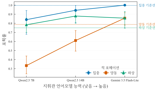
Figure 18: 지휘관 능력 사다리(기동 계층은 휴리스틱으로 고정). 점선과 오른쪽 이름표는 같은 포메이션의 휴리스틱 배정 기준선이고, 오차막대는 시드 부트스트랩 95% 신뢰구간이다. 관건은 성능이 오르는지가 아니라 어디에서 기준선을 교차하는가이다 — 양동 포메이션에서 7B와 14B는 기준선 아래에 있고 Gemini 에서 처음 위로 올라선다. 집중 포메이션은 기준선이 0.997로 천장이지만 세 모델이 거기 붙어 있는 것은 아니다 — Gemini만 기준선에 닿고, 7B는 0.840으로 기준선보다 유의하게 낮다. 천장은 개선했지만 여지를 없앨 뿐 악화여지를 없애지 않는다($6.2).
