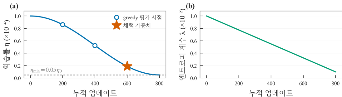
Figure 13: 학습 코드가 실제로 쓴 스케줄. (a) 식 (42)의 단일 주기 코사인 학습률. 원 표식은 200 업데이트마다의 greedy 평가 시점, 별표는 채택 가중치(600 업데이트, \eta_t \approx 1.9 \times 10^{-5} ), 회색 파선은 \eta_{\min} 이다. (b) 엔트로피 계수 \lambda_H(t) 의 선형 감쇠 ( 0.01 \rightarrow 0.001 ).
