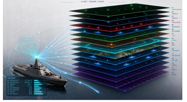
Figure 4: 15채널 관측의 구성. 전역 9채널(01–09), 방어정별 3채널(10–12), 좌표 3채널(13–15)이 같은 격자에 겹쳐 하나의 다채널 영상을 이룬다. 오른쪽의 채널 이름은 구현의 이름과 같다. 왼쪽 아래는 격자에 담기지 않고 벡터로 들어가는 방어정 자체 상태 \mathbf{o}_p \in \mathbb{R}^8 — 위치 2, heading 단위벡터 2, 잔여 그물 1, 전개 중 여부 1, 배정 요격점 2이며, 요격점 두 성분은 배정이 없으면 0이다. 그림의 좌측 시선원뿔(“egocentric FOV”)과 함정 형상은 삽화의 표현이다 — 본 연구의 래스터는 방어정 시야가 아니라 모선을 중앙에 둔 전역 격자이며, 방어정마다 달라지는 것은 3채널(10–12)과 \mathbf{o}_p 뿐이다.
