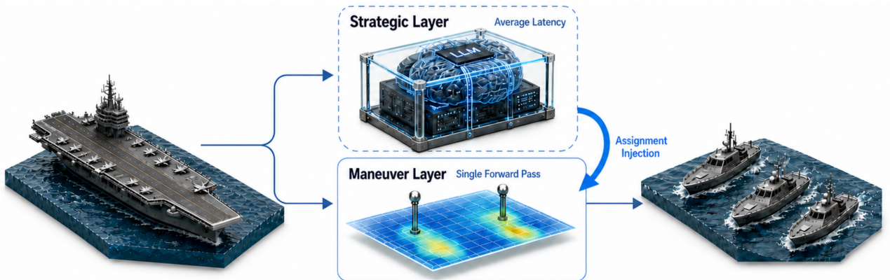
Figure 2: 속도가 다른 2계층 비동기 구조. 두 판단 계층은 25초마다 결정을 내리지만, 전략 계층(언어모델 지휘관)은 로컬 14B 모델에서 평균 16.6초가 걸리는 반면 기동 계층의 순전파 시간은 무시할 수 있다. 그래서 전략 계층 호출만 비동기로 분리하고, 저수준 제어(PD 조타)는 1초 주기로 돈다.
