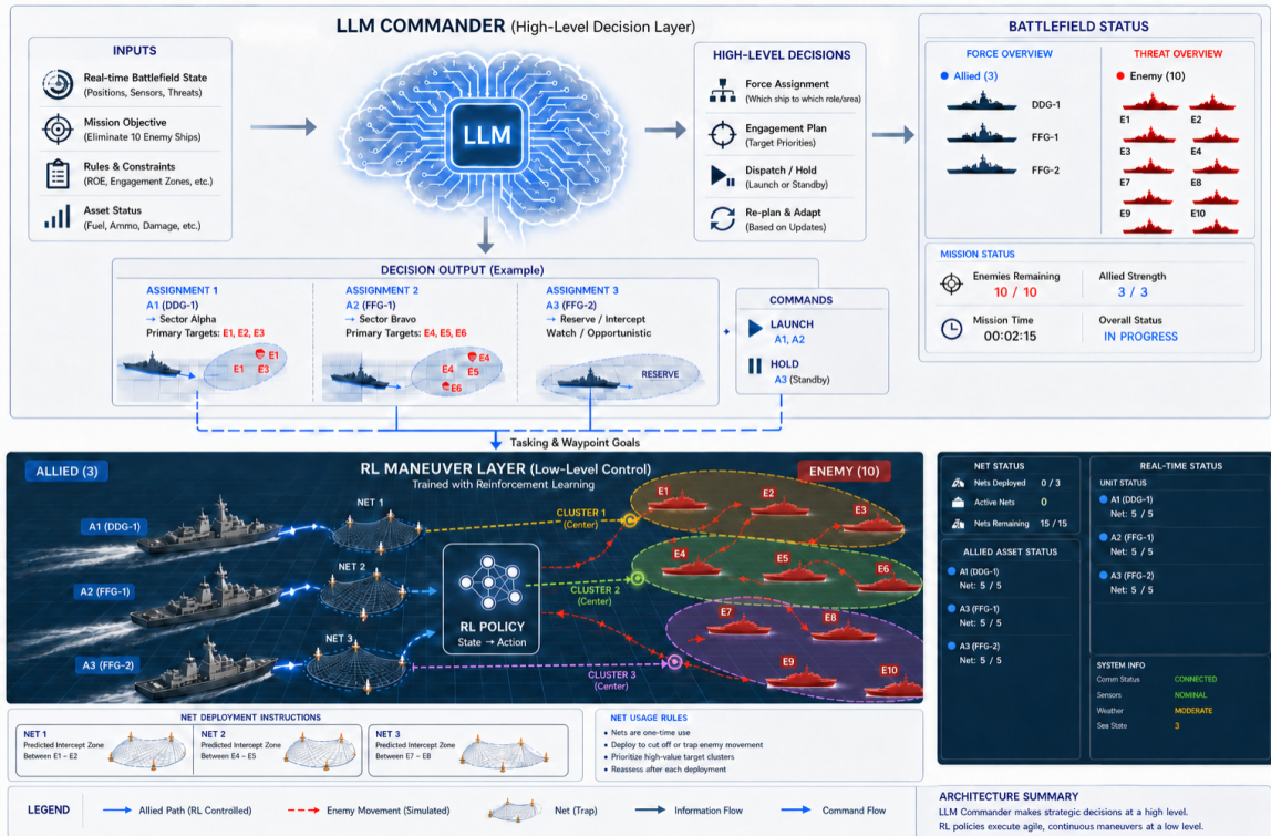
Figure 1: 제안 체계의 개요. 위: 전략 계층 — 언어모델 지휘관이 전장 상태·임무 목표·교전 규칙·자산 상태를 입력받아 어느 방어정이 어느 무리를 맡는가(배정)와 대기 여부를 구조화된 출력으로 낸다. 아래: 기동 계층 — 배정을 조건으로 학습된 정책이 각 방어정의 그물벽 위치(경유점 두 개)를 정한다. 방어정은 적선보다 느리므로 추격 대신 접근 회랑을 앞질러 그물벽으로 차단한다. 그림의 합성 형상과 패널은 개념 전달용 삽화이며, 실제 입출력 형식은 §4에 정의한다.
