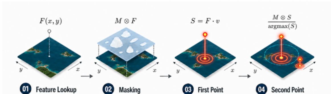
Figure 9: 점수맵 위 픽셀 지목의 네 단계. ① 복호기가 낸 픽셀별 특징 F(x, y) . ② 유효 마스크 M 을 곱해 놓을 수 없는 칸을 차단한다 (§4.4.3). ③ 질의 \mathbf{v} 와의 내적으로 점수맵 S = F \cdot \mathbf{v} 를 얻고 최대 칸을 첫 점으로 고른다. ④ 첫 점의 특징을 질의에 더해( \mathbf{q} \leftarrow \mathbf{q} + \mathbf{f}_0 ) 같은 절차로 두 번째 점을 고르되, 첫 점과의 간격 상·하한(파선 원)을 마스크에 추가한다. 두 점을 잇는 선분이 그물벽이다.
