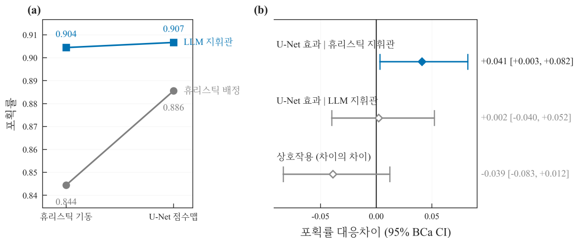
Figure 17: 2 × 2 상호작용(지휘관 = Gemini 3.5 Flash-Lite). (a) 네 셀의 포획률 평균. 두 선이 평행에 가까울수록 두 계층의 기여가 가산적이다. (b) 이 논문이 실제로 검정한 양 — 시드 대응차이 세 가지와 그 BCa 95 % 신뢰구간. 속이 빈 표식은 구간이 0 을 포함한다. (a)에 오차막대를 두지 않은 것은 의도적이다 — 셀별 구간은 대응이 풀린 구간이라 시나리오 난이도의 분산을 그대로 포함해 넓고, 그것을 겹쳐 그리면 유의한 대응차이가 유의하지 않은 것처럼 읽힌다. 불확실성은 전부 (b)에 있다.
