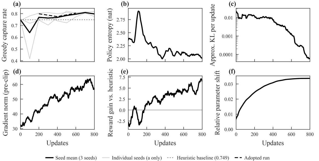
Figure 12: 수렴 진단 — 채택 런과 같은 설정을 시드 3개로 다시 돌린 학습 동역학. 검정 굵은 선은 시드 평균(40 업데이트 이동평균)이며, 시드별 꺾은선은 (a)에만 연회색으로 두었다. (a) 100 업데이트마다의 greedy 포획률(연회색은 시드별, 검정 실선은 평균, 검정 파선은 채택 런, 점선은 같은 프로토콜로 랜 휴리스틱 기준선 0.749). (b) 1단계 픽셀 분포의 엔트로피. 유효 픽셀 중앙값 273개의 균일분포 상한은 \ln 273 \approx 5.6 \text{ nat} 로 추 밖에 있다. (c) 갱신 전후 정책의 근사 KL 발산(같은 관측·같은 표본 후보, 로그측). (d) 클리핑 전 그래디언트 노름 — 800 업데이트 내내 클립 한계 1.0의 수십 배라 수렴 지표가 아니다. (e) 표본 후보 보상에서 휴리스틱 후보 보상을 뺀 값. 0 을 넘으면 정책의 표본이 휴리스틱을 앞선다. (f) 행동복제 초기점으로부터의 상대 파라미터 이동 거리.
