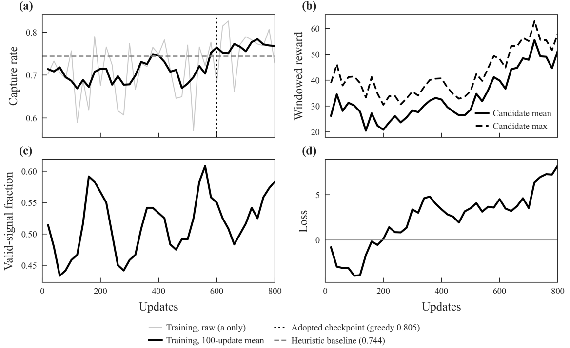
Figure 11: GRPO 학습 경과( 50^2 격자, 후보 G = 8 , 후보 평가 구간 180 step, 실해역 6곳 로테이션(Fig. 6), 800 업데이트). 검정 굵은 선은 20 업데이트마다 기록한 원자료의 100 업데이트 이동평균이며, (a)에만 원자료를 연회색 가는 선으로 함께 두었다. (a) 포획률(Capture rate). 200 업데이트마다의 greedy 평가는 0.799, 0.775, 0.805 였고, 파선은 휴리스틱 기준선 0.744이다. 세로 점선(600 업데이트, greedy 0.805) 이 본 논문이 평가하는 가중치이다. (b) 후보 평균 보상(실선)과 후보 최대 보상(파선) — 둘의 간격이 그룹 내 변별력이다. (c) 후보 간 분산이 0이 아닌 월드의 비율(Valid-signal fraction; 학습 신호가 실제로 생긴 비율). (d) 손실(정책경사 + 엔트로피). 부호와 크기 자체는 수렴 지표가 아니다.
