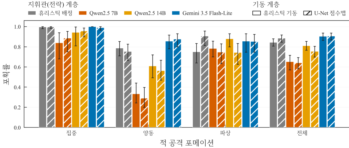
Figure 15: 포메이션 × 조건 포획률. 색은 전략 계층(지휘관), 빛금은 기동 계층을 나타내며, 같은 색 안에서 인접한 두 막대가 곧 그 지휘관에서의 U-Net 효과이다. 무채색 두 막대는 언어모델을 쓰지 않는 기준선이고, 그 오른쪽부터가 언어모델 지휘관이며 모델 규모 오름차순으로 놓았다 — 성능 순서가 아니다. 실제로 7B는 기준선보다 낮다($6.5). 오차막대는 표준편차가 아니라 시드 부트스트랩 95 % 신뢰구간이다. 집중 포메이션에서 여덟 조건이 모두 상단에 몰려 있는 것이 천장 효과이며($6.2), 양동 포메이션에서만 지휘관 능력축이 넓게 벌어진다.
