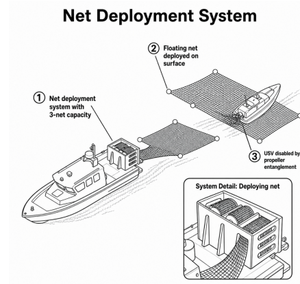
Figure 3: 후미 투하식 부유 그물에 의한 포획 개념 — 그물 위를 지나가는 적 USV의 프로펠러가 얽혀 추진을 잃는다.
