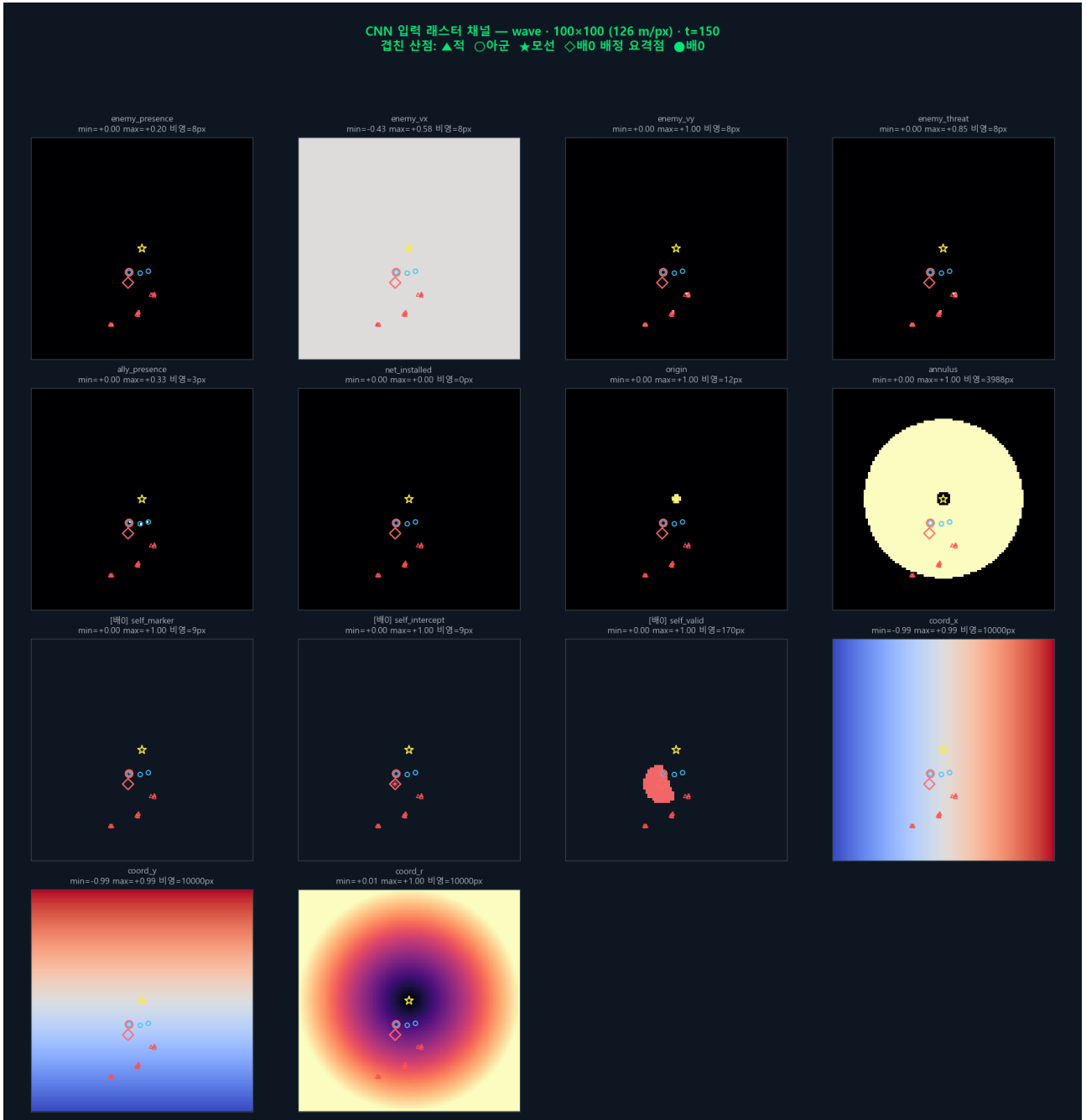
Figure 5: 래스터화된 다채널 관측의 채널별 분해. 전역 채널(적 밀도, 적 진행 x \cdot y , 적 위협도, 아군 위치, 설치된 그물, 원점, 요격 환경), 방어정별 채널(자기 위치, 배경 요격점, 유효 영역), 좌표 채널( x, y, r )이 같은 격자에 정렬된다. 각 패널에 min/max와 비영 픽셀 수를 함께 표시하였다. 이 그림은 시각적 판독을 위해 100 \times 100 (126 m/px)로 렌더하였다 — 본문의 학습·평가 설정은 50 \times 50 (252 m/px)이며 채널 구성과 의미는 동일하다. 육지 채널은 이 장면에 육지가 없어 표시되지 않았다.
