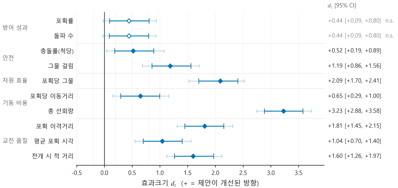
Figure 18: 제안(11m_unet@Gemini) 대 기준선(heur_heur)의 전 지표 효과크기. 마름모가 점추정이고, 굵은 선이 95 % 신뢰 구간, 그 바깥의 얇은 선이 지표 10개에 대한 Bonferroni 보정 구간(99.5 %)이다. 속이 찬 표식은 보정 구간까지 0을 배제한 지표이며, 속이 빈 표식은 보정 구간을 넘지 못해 n.s.로 적었다 — Table 8의 단검 표시와 같은 판정이다. 부호는 개선 방향이 항상 양수가 되도록 통일하였다(낮을수록 좋은 지표는 뒤집었다). d_z 의 구간은 평균차의 BCa 신뢰구간을 sd(d) 로 나눈 것이므로, 이 그림이 0을 배제하는 것과 Table 8의 평균차 구간이 0을 배제하는 것은 같은 사건이다. 포획률의 효과크기가 10개 지표 중 최하위권이라는 점이 이 그림의 요지이다.
