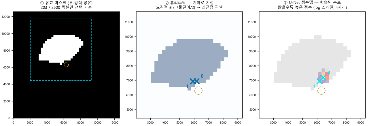
Figure 3: 기동 계층 두 방식의 비교(학습된 체코포인트의 실제 출력, 같은 전장·같은 시점). 왼쪽: 두 방식이 공유하는 유효 마스크 — 2500칸 중 203칸만 선택 가능하다. 가운데: 휴리스틱은 유효 영역 안에서 기하로 정해진 두 점을 지목하며, 나머지 칸에 대한 선호를 표현하지 않는다(영역 전체가 균일하게 칠해져 있다). 오른쪽: 점수맵 정책은 같은 영역 위에 학습된 분포를 얹어 소수의 칸에 확률을 집중시킨다. 두 방식은 같은 격자·같은 마스크·같은 거리 제약을 통과한다 — 행동공간이 동일해야 성능 차이가 방법의 차이가 된다.
