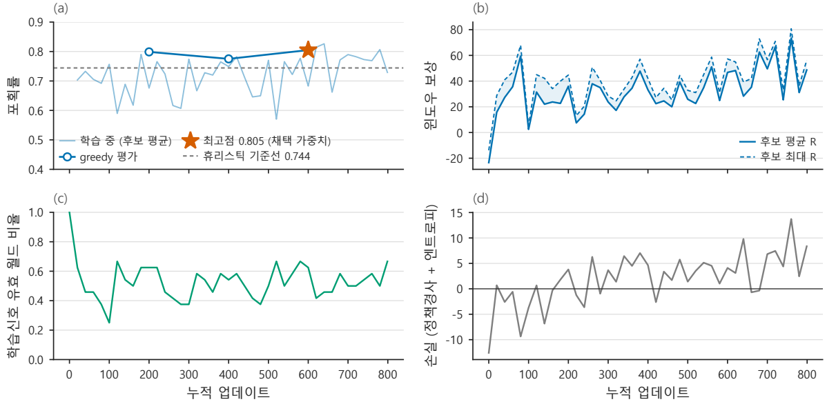
Figure 14: GRPO 학습 경과(50 2 격자, 후보 G = 8 , 후보 평가 구간 180 step, 실해역 6곳 로테이션(Fig. 12), 800 업데이트). (a) 포획률. 엷은 선은 학습 중 후보 평균, 원 표식은 200 업데이트마다의 greedy 평가, 회색 파선은 휴리스틱 기준선 0.744이다. 별표(600 업데이트, 0.805)가 본 논문이 평가하는 가중치이다. (b) 후보 평균 보상과 후보 최대 보상 — 둘의 간격이 그룹 내 변별력이다. (c) 후보 간 분산이 0이 아닌 월드의 비율(학습 신호가 실제로 생긴 비율). (d) 손실(정책경사 + 엔트로피). 부호와 크기 자체는 수렴 지표가 아니다.
