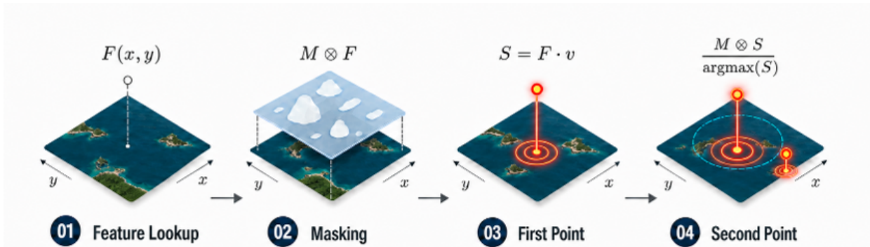
Figure 10: 점수맵 위 픽셀 지목의 네 단계. ① 복호기가 낸 픽셀별 특징 F(x, y) . ② 유효 마스크 M 을 곱해 놓을 수 없는 칸을 차단한다 (§4.3.3). ③ 질의 \mathbf{v} 와의 내적으로 점수맵 S = F \cdot \mathbf{v} 를 얻고 최대 칸을 첫 점으로 고른다. ④ 첫 점의 특징을 질의에 더해( \mathbf{q} \leftarrow \mathbf{q} + \mathbf{f}_0 ) 같은 절차로 두 번째 점을 고르되, 첫 점과의 간격 상·하한(파선 원)을 마스크에 추가한다. 두 점을 잇는 선분이 그물벽이다.
