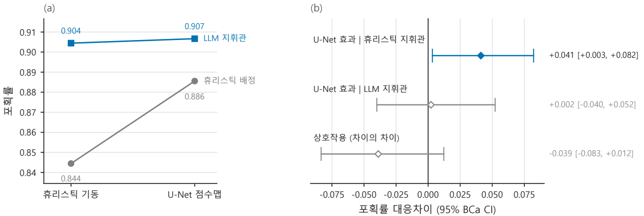
Figure 19: 2 × 2 상호작용(지휘관 = Gemini 3.5 Flash-Lite). (a) 네 셀의 포획률 평균. 두 선이 평행에 가까울수록 두 계층의 기여가 가산적이다. (b) 이 논문이 실제로 검정한 양 — 시드 대응차이 세 가지와 그 BCa 95 % 신뢰구간. 속이 빈 표식은 구간이 0 을 포함한다. (a)에 오차막대를 두지 않은 것은 의도적이다 — 셀별 구간은 대응이 풀린 구간이라 시나리오 난이도의 분산을 그대로 포함해 넓고, 그것을 겹쳐 그리면 유의한 대응차이가 유의하지 않은 것처럼 읽힌다. 불확실성은 전부 (b)에 있다.
