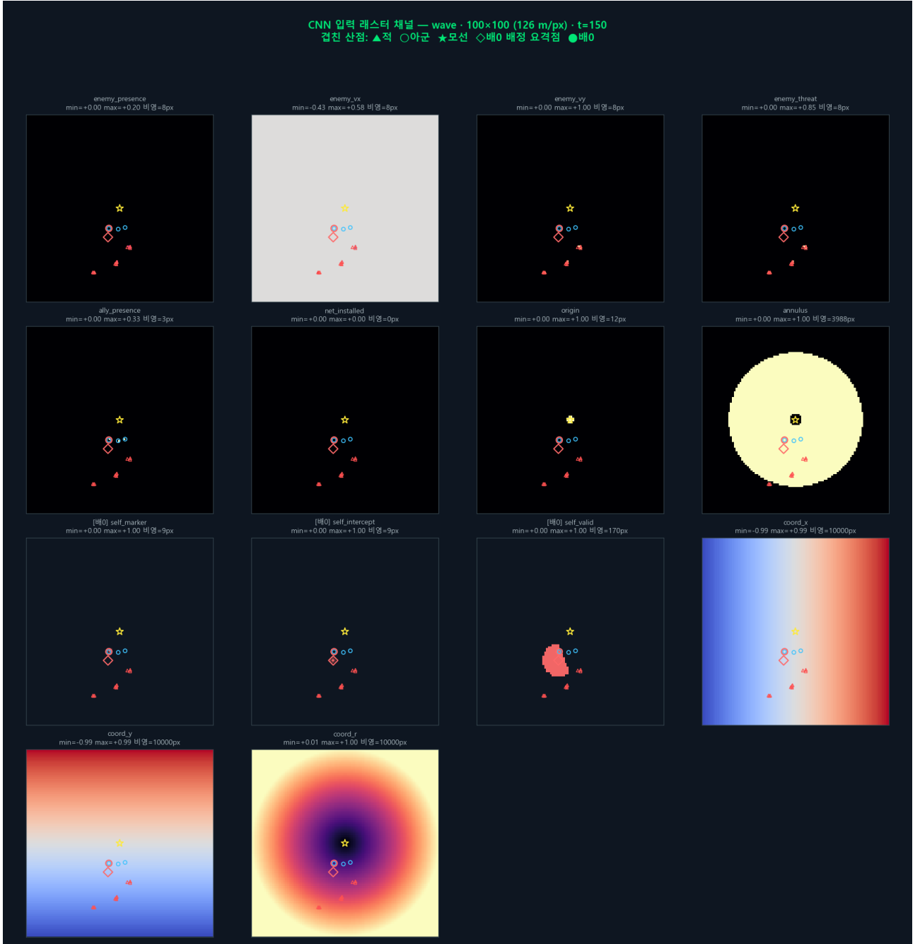
Figure 5: 래스터화된 다채널 관측의 채널별 분해. 전역 채널(적 밀도, 적 진행 x \cdot y , 적 위협도, 아군 위치, 설치된 그물, 원점, 요격 현황), 방어정별 채널(자기 위치, 배정 요격점, 유효 영역), 좌표 채널( x, y, r )이 같은 격자에 정렬된다. 각 패널에 min/max와 비영 픽셀 수를 함께 표시하였다. 이 그림은 시각적 판독을 위해 100 \times 100 ( 126 \text{ m/px} )로 렌더하였다 — 본문의 학습·평가 설정은 50 \times 50 ( 252 \text{ m/px} )이며 채널 구성과 의미는 동일하다. 육지 채널은 이 장면에 육지가 없어 표시되지 않았다.
