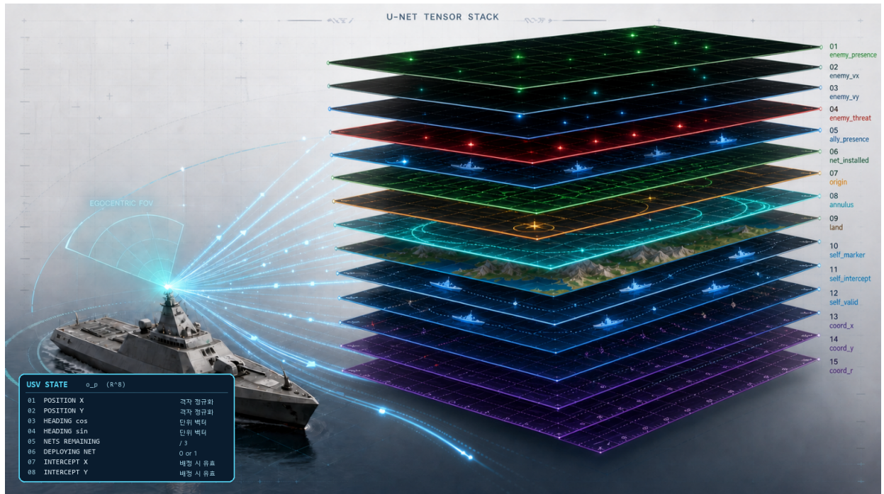
Figure 4: 15채널 관측의 구성. 전역 9채널(01–09), 방어정별 3채널(10–12), 좌표 3채널(13–15)이 같은 50 × 50 격자에 겹쳐 하나의 다채널 영상을 이룬다. 오른쪽의 채널 이름은 구현의 이름과 같다. 왼쪽 아래는 격자에 담기지 않고 벡터로 들어가는 방어정 자체 상태 \mathbf{o}_p \in \mathbb{R}^8 — 위치 2, heading 단위벡터 2, 잔여 그물 1, 전개 중 여부 1, 배정 요격점 2이며, 요격점 두 성분은 배정이 없으면 0이다. 그림의 좌측 시선원뿔(“egocentric FOV”)과 함정 형상은 삽화의 표현이다 — 본 연구의 래스터는 방어정 시야가 아니라 모션을 중앙에 둔 전역 격자이며, 방어정마다 달라지는 것은 3채널(10–12)과 \mathbf{o}_p 뿐이다.
