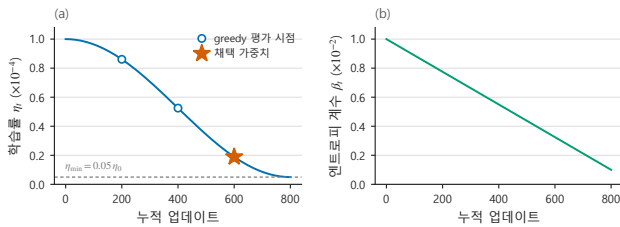
Figure 16: 학습 코드가 실제로 쓴 스케줄. (a) 식 (38)의 단일 주기 코사인 학습률. 원 표식은 200 업데이트마다의 greedy 평가 시점, 별표는 채택 가중치(600 업데이트, \eta_t \approx 1.9 \times 10^{-5} ), 회색 파선은 \eta_{\min} 이다. (b) 엔트로피 계수 \lambda_H(t) 의 선형 감쇠 ( 0.01 \rightarrow 0.001 ).
