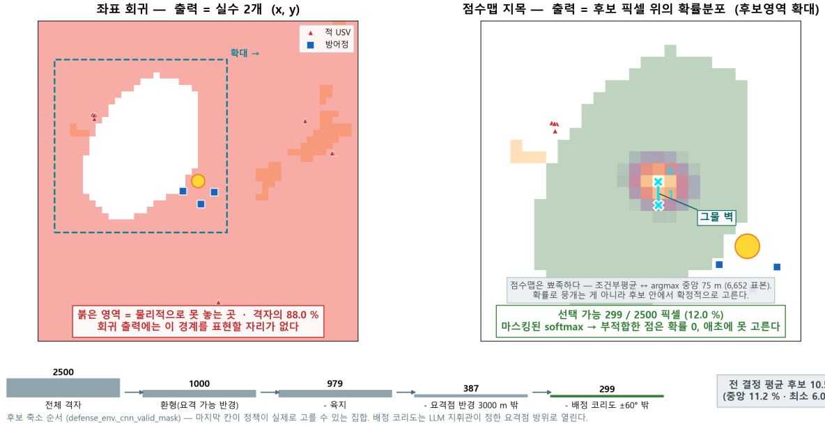
Figure 9: 왜 좌표 회귀가 아니라 점수맵 위 픽셀 지목인가(학습된 체크포인트의 실제 출력). 왼쪽: 연속 좌표를 회귀하는 출력에는 “놓을 수 없는 곳”을 표현할 자리가 없다 — 이 장면에서 붉은 영역이 격자의 88.0%다. 오른쪽: 같은 장면을 후보 영역으로 확대한 점수 분포와 선택된 두 픽셀, 그리고 그 둘을 잇는 그물벽이다. 마asking된 softmax 아래에서 부적합한 칸은 확률이 0이라 애초에 선택되지 않는다. 아래 막대: 제약이 순차 적용되며 후보가 줄어드는 과정이다 (2500 → 1000 → 979 → 387 → 299, 12.0%). 전 결정 평균 후보는 10.5%였다.
