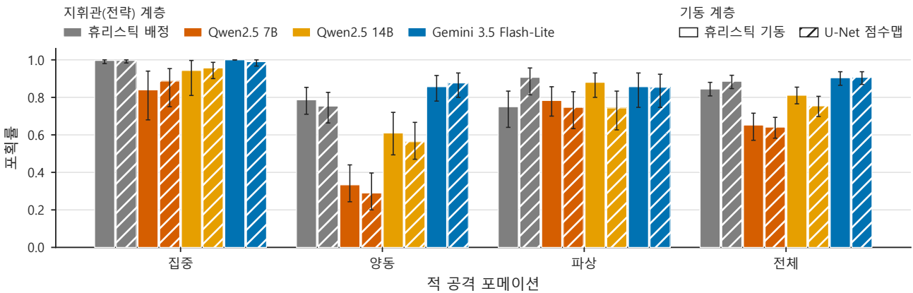
Figure 17: 포메이션 × 조건 포획률. 색은 전략 계층(지휘관), 빗금은 기동 계층을 나타내며, 같은 색 안에서 인접한 두 막대가 곧 그 지휘관에서의 U-Net 효과이다. 무채색 두 막대는 언어모델을 쓰지 않는 기준선이고, 그 오른쪽부터가 언어모델 지휘관이며 모델 규모 오름차순으로 놓았다 — 성능 순서가 아니다. 실제로 7B는 기준선보다 낮다($6.6). 오차막대는 표준편차가 아니라 시드 부트스트랩 95 % 신뢰구간이다. 집중 포메이션에서 여덟 조건이 모두 상단에 몰려 있는 것이 천장 효과이며($6.3), 양동 포메이션에서만 지휘관 능력축이 넓게 벌어진다.
