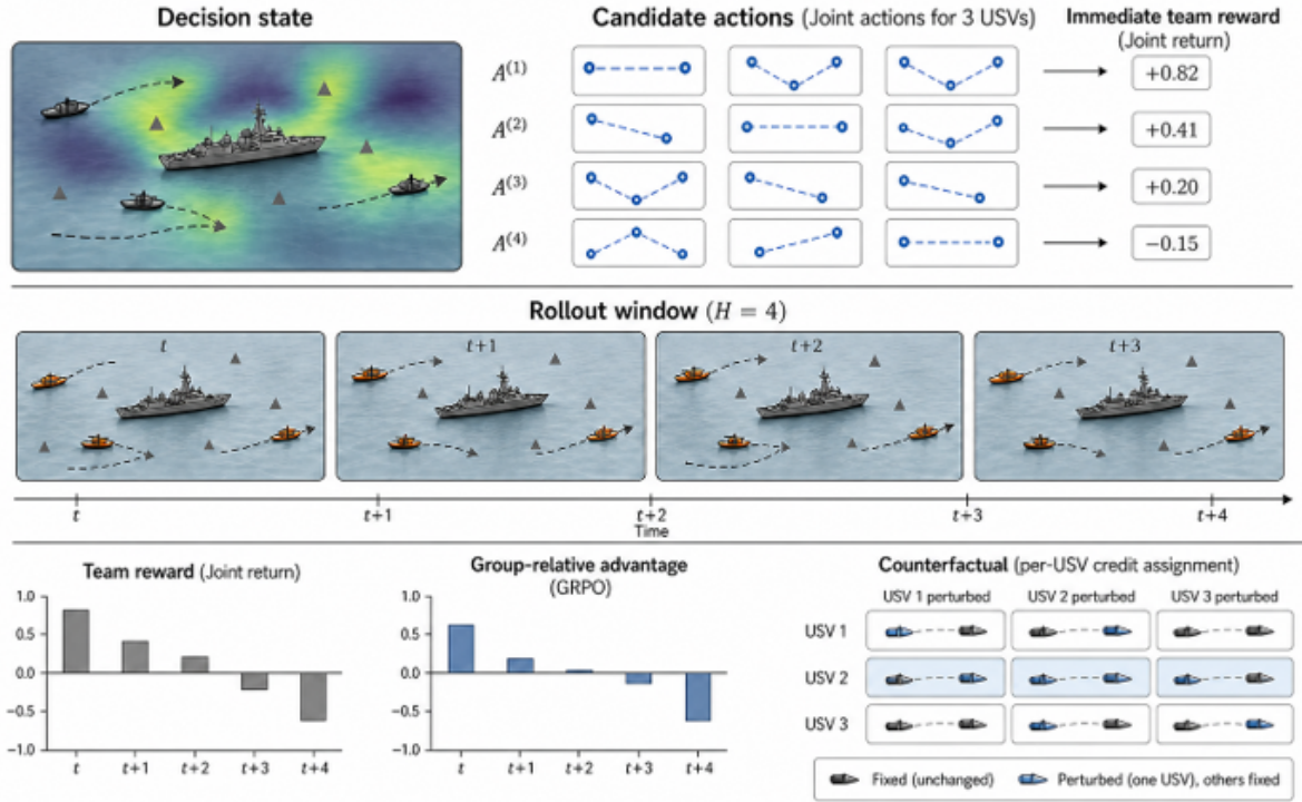
Figure 11: 가치망 없는 다중 방어정 그룹 상대 최적화의 한 갱신. 위: 한 결정 상태에서 G 개의 결합 행동 후보를 표집하고, 각 후보를 시뮬레이터에서 공통 구간만큼 실제로 진행시켜 팀 보상을 얻는다. 가운데: 후보 평가에 쓰이는 롤아웃 창. 아래 왼쪽·가운데: 팀 보상을 후보 간 상대 비교로 이득으로 바꾼다 (식 (22)). 아래 오른쪽: 반사실적 크레딧 — 한 척의 행동만 바꾸고 나머지는 고정된 채 시뮬레이터를 다시 진행시켜, 그 차이를 그 배의 몫으로 돌린다 (§4.4; 구현된 변형이며 채택 런은 팀 이득 손실을 썼다). 그림은 기전 전달을 위해 후보 수와 창을 G = 4 , H = 4 로 줄여 그렸으며 실제 학습은 G = 8 , 평가 구간 180 step 이다.
