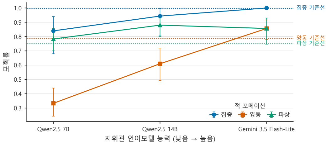
Figure 20: 지휘관 능력 사다리(기동 계층은 휴리스틱으로 고정). 점선과 오른쪽 이름표는 같은 포메이션의 휴리스틱 배정 기준선이고, 오차막대는 시드 부트스트랩 95 % 신뢰구간이다. 판건은 성능이 오르는지가 아니라 어디에서 기준선을 교차하는 가이다 — 양동 포메이션에서 7B와 14B는 기준선 아래에 있고 Gemini 에서 처음 위로 올라선다. 집중 포메이션은 기준선이 0.997로 천장이지만 세 모델이 거기 붙어 있는 것은 아니다 — Gemini만 기준선에 닿고, 7B는 0.840으로 기준선보다 유의하게 낮다. 천장은 개선 여지를 없앨 뿐 악화 여지를 없애지 않는다($6.3).
