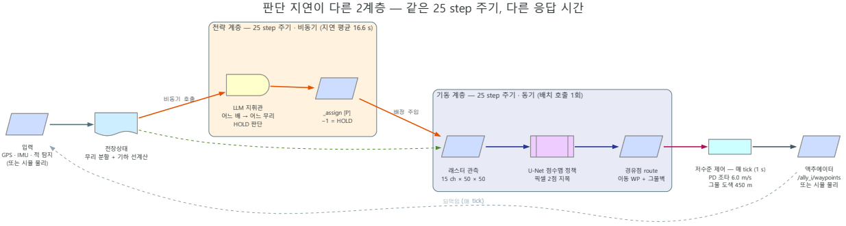
Figure 2: 2계층 비동기 구조와 갱신 주기. 두 판단 계층은 같은 결정 주기 (25 step = 25초)로 갱신되지만 응답 지연이 다르다 — 전략 계층은 로컬 14B 모델에서 평균 16.6초로 주기의 3분의 2를 소모하는 반면, 기동 계층의 순전파 시간은 그에 비해 무시할 수 있다. 그래서 전략 계층 호출만 비동기로 분리한다. 저수준 제어(PD 조타)는 그보다 25배 빠른 1초 주기로 돈다.
