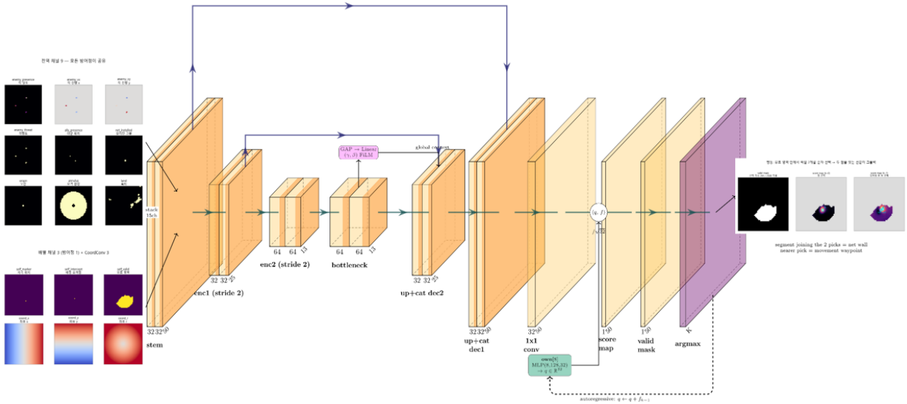
Figure 8: 기동 계층의 텐서 흐름(구현 참조도, 244,389 파라미터, d = 32 , K = 2 ). 왼쪽: 실제 관측 15채널 — 전역 9채널 (위)과 방어정별 3채널 + CoordConv 3채널(아래)의 학습된 체크포인트 출력 화면. 가운데: stem \rightarrow enc1 \rightarrow enc2(stride 2) \rightarrow bottleneck \rightarrow dec2 \rightarrow dec1의 U-Net. 병목에서 전역 평균 풀링 \rightarrow 선형층으로 FiLM 계수 (\gamma, \beta) 를 만들어 병목 특징을 변조하고, 방어정 자체 상태 \mathbf{o}_p \in \mathbb{R}^8 은 MLP( 8 \rightarrow 128 \rightarrow 32 )를 거쳐 질의 q 가 된다. 스킵 연결은 위쪽 파란 화살표. 오른쪽: 1 \times 1 합성곱으로 픽셀 특징 f 을 내고, 질의 q 와의 내적 \langle q, f \rangle / \sqrt{d} 로 점수맵을 만든 뒤 유효 마스크를 거쳐 argmax로 K = 2 픽셀을 고른다. 아래 점선은 자기회귀 q \leftarrow q + f_{k-1} — 첫 점의 특징을 질의에 더해 두 번째를 고른다. 본문 Fig. 7는 같은 구조의 개념 일러스트이고, 이 그림은 형상과 조건화 지점을 정확히 적은 판이다.
