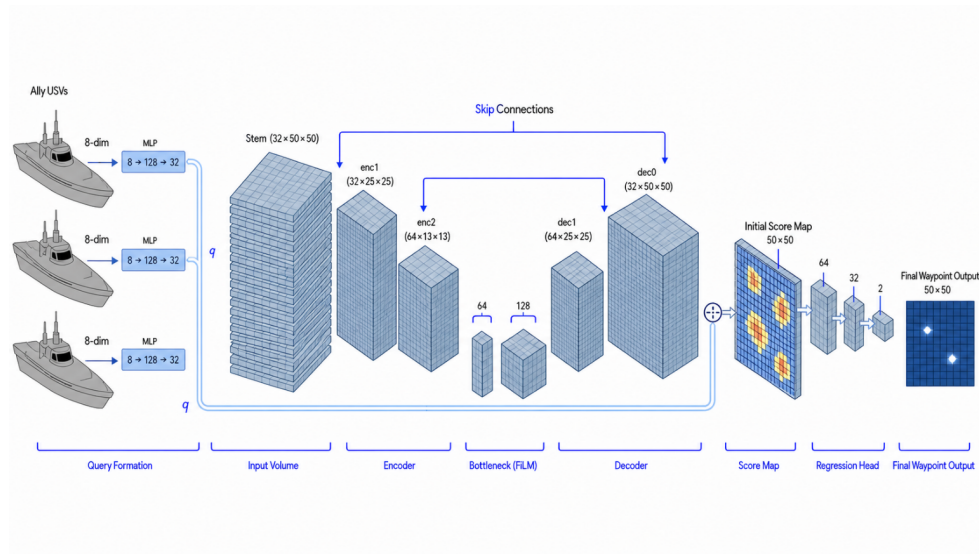
Figure 7: 점수맵 정책의 구조. 각 방어정의 8차원 상태가 공유 MLP( 8 \rightarrow 128 \rightarrow 32 )를 지나 질의 q 가 되고, 15채널 관측은 Stem( 32 \times 50 \times 50 ) – 인코더( 32 \times 25 \times 25 \rightarrow 64 \times 13 \times 13 ) – FiLM 병목 – 디코더( 64 \times 25 \times 25 \rightarrow 32 \times 50 \times 50 )를 지난다. skip 연결이 인코더의 위치 정보를 디코더로 전달한다. 질의와 픽셀 특징의 내적이 50 \times 50 점수맵을 이루고, 회귀 머리가 선택된 칸 안의 부화소 오프셋 2개를 낸다. 방어정을 배치 축으로 쌓아 결정당 한 번의 배치 호출로 통과하며 (그림의 입력 부피는 방어정마다 하나씩이다), 가중치는 전 방어정이 공유하므로 모델 크기는 방어정 수에 불변이다.
