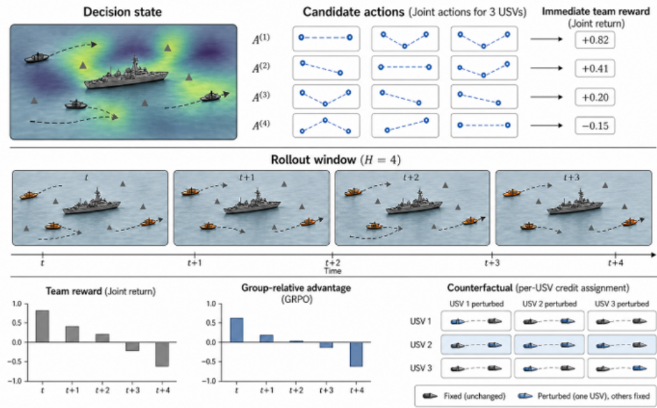
Figure 11: 가치망 없는 다중 방어정 그룹 상대 최적화의 한 갱신. 위: 한 결정 상태에서 G 개의 결합 행동 후보를 표집하고, 각 후보를 시뮬레이터에서 공통 구간만큼 실제로 진행시켜 팀 보상을 얻는다. 가운데: 후보 평가에 쓰이는 롤아웃 창. 아래 왼쪽·가운데: 팀 보상을 후보 간 상대 비교로 이득으로 바꾼다 (식 (9)). 아래 오른쪽: 반사실적 크레딧 — 한 척의 행동만 바꾸고 나머지는 고정한 채 시뮬레이터를 다시 진행시켜, 그 차이를 그 배의 몫으로 돌린다 (§4.4). 그림은 기전 전달을 위해 후보 수와 창을 G = 4 , H = 4 로 줄여 그렸으며 실제 학습은 G = 8 , 평가 구간 180 step이다.
