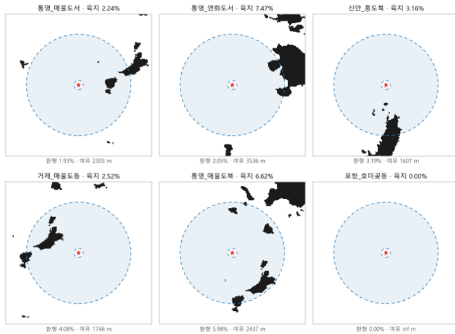
Figure 12: 학습에 쓴 실해역 6곳의 육지 마스크(Fig. 6의 절차를 각 해역에 적용한 결과, 12.6km 박스). 별표는 모선, 파선 원은 요격 환형이다. 각 패널 위의 백분율은 박스 안 육지 비율, 아래는 요격 환형에 육지가 잠식한 비율과 모선에서 가장 가까운 육지까지의 여유 거리이다. 오른쪽 아래(포항 호미곶 동측)는 육지가 없는 외해로, 지형이 없는 상황을 학습 분포에 넣기 위한 대조 해역이다.
