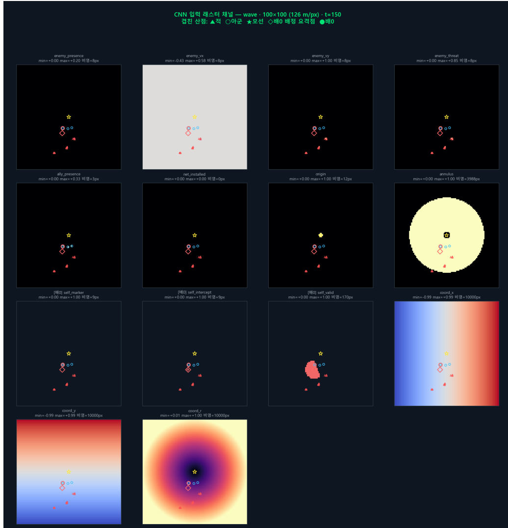
Figure 5: 래스터화된 다채널 관측의 채널별 분해. 전역 채널(적 밀도, 적 진행 x, y , 적 위협도, 아군 위치, 설치된 그물, 원점, 요격 환경), 방어정별 채널(자기 위치, 배정 요격점, 유효 영역), 좌표 채널( x, y, r )이 같은 격자에 정렬된다. 각 패널에 min/max와 비영 픽셀 수를 함께 표시하였다. 이 그림은 시각적 판독을 위해 100 \times 100 (126 m/px)로 렌더하였다 — 본문의 학습·평가 설정은 50 \times 50 (252 m/px)이며 채널 구성과 의미는 동일하다. 육지 채널은 이 장면에 육지가 없어 표시되지 않았다.
