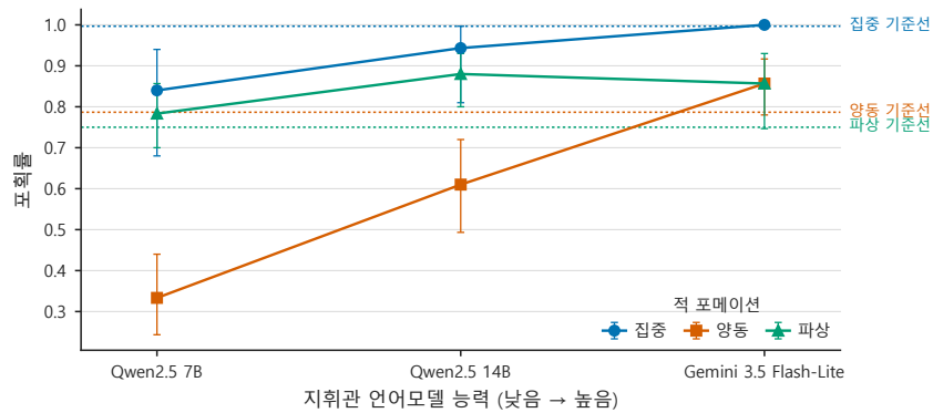
Figure 20: 지휘관 능력 사다리(기동 계층은 휴리스틱으로 고정). 점선과 오른쪽 이름표는 같은 포메이션의 휴리스틱 배정 기준선이고, 오차막대는 시드 부트스트랩 95 % 신뢰구간이다. 관건은 성능이 오르는지가 아니라 어디에서 기준선을 교차하는가이다 — 양동 포메이션에서 7B와 14B는 기준선 아래에 있고 Gemini 에서 처음 위로 올라선다. 집중 포메이션은 기준선이 0.997로 천장이지만 세 모델이 거기 붙어 있는 것은 아니다 — Gemini만 기준선에 닿고, 7B는 0.840으로 기준선보다 유의하게 낮다. 천장은 개선 여지를 없앨 뿐 악화 여지를 없애지 않는다(§6.3).
