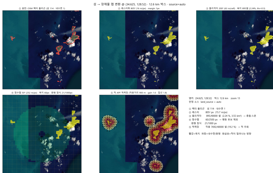
Figure 6: 실해역 지형의 반영 과정(통영 매물도 인근, 12.6km 박스). ① OpenStreetMap 벡터 폴리곤 → ② 고해상도 래스터(805 2 , 16 m/px) → ③ 충돌 판정용 물리 격자(200 2 , 63 m/cell) → ④ 정책 격자(50 2 , 252 m/px)로 면적비 다운샘플. 판정과 관측을 다른 해상도로 두는 이유는 충돌은 이진 판정을 요구하고, 관측은 해안선이 계단으로 들어가면 안 되기 때문이다. ⑤는 적의 우회를 유도하는 척력장으로, 관측이 아니라 적 기동 모형의 일부다.
