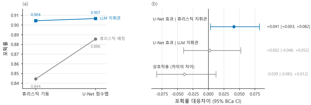
Figure 19: 2 \times 2 상호작용(지휘관 = Gemini 3.5 Flash-Lite). (a) 네 셀의 포획률 평균. 두 선이 평행에 가까울수록 두 계층의 기여가 가산적이다. (b) 이 논문이 실제로 검정한 양 — 시드 대응차이 세 가지와 그 BCa 95 % 신뢰구간. 속이 빈 표식은 구간이 0 을 포함한다. (a) 에 오차막대를 두지 않은 것은 의도적이다 — 셀별 구간은 대응이 풀린 구간이라 시나리오 난이도의 분산을 그대로 포함해 넓고, 그것을 겹쳐 그리면 유의한 대응차이가 유의하지 않은 것처럼 읽힌다. 불확실성은 전부 (b)에 있다.
