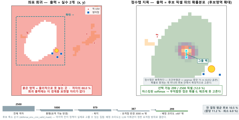
Figure 9: 왜 좌표 회귀가 아니라 점수맵 위 픽셀 지목인가(학습된 체크포인트의 실제 출력). 왼쪽 : 연속 좌표를 회귀하는 출력에는 “놓을 수 없는 곳”을 표현할 자리가 없다 — 이 장면에서 붉은 영역이 격자의 88.0%다. 오른쪽 : 같은 장면을 후보 영역으로 확대한 점수 분포와 선택된 두 픽셀, 그리고 그 둘을 잇는 그물벽이다. 마스킹된 softmax 아래에서 부적합한 칸은 확률이 0이라 애초에 선택되지 않는다. 아래 막대 는 제약이 순차 적용되며 후보가 줄어드는 과정이다 (2500 → 1000 → 979 → 387 → 299, 12.0%). 전 결정 평균 후보는 10.5%였다.
