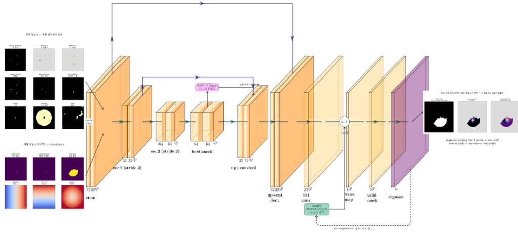
Figure 8: 기동 계층의 텐서 흐름(구현 참조도, 244,389 파라미터, d = 32 , K = 2 ). 왼쪽 : 실제 관측 15채널 — 전역 9채널(위)과 방어정별 3채널 + CoordConv 3채널(아래)의 학습된 체크포인트 출력 화면. 가운데 : stem \rightarrow enc1 \rightarrow enc2(stride 2) \rightarrow bottleneck \rightarrow dec2 \rightarrow dec1 의 U-Net. 병목에서 전역 평균 풀링 \rightarrow 선형층으로 FiLM 계수 (\gamma, \beta) 를 만들어 방어정 자체 상태 \mathbf{o}_p \in \mathbb{R}^8 (MLP 8 \rightarrow 128 \rightarrow 32 )로 조건화한다. 스킵 연결은 위쪽 파란 화살표. 오른쪽 : 1 \times 1 합성곱으로 픽셀 특징 f 를 내고, 질의 q 와의 내적 \langle q, f \rangle / \sqrt{d} 로 점수맵을 만든 뒤 유효 마스크를 거쳐 argmax로 K = 2 픽셀을 고른다. 아래 점선은 자기회귀 q \leftarrow q + f_{k-1} — 첫 점의 특징을 질의에 더해 두 번째를 고른다. 본문 Fig. 7는 같은 구조의 개념 일러스트이고, 이 그림은 형상과 조건화 지점을 정확히 적은 판이다.
