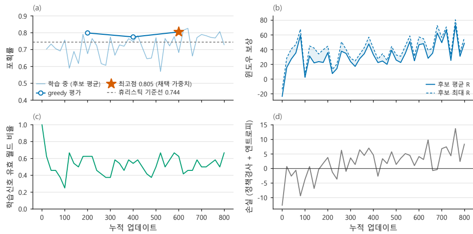
Figure 14: GRPO 학습 경과( 50^2 격자, 후보 G = 8 , 후보 평가 구간 180step, 실패역 6곳 로테이션(Fig. 12), 800 업데이트). (a) 포획률. 얇은 선은 학습 중 후보 평균, 원 표식은 200 업데이트마다의 greedy 평가, 회색 파선은 휴리스틱 기준선 0.744이다. 별표(600 업데이트, 0.805) 가 본 논문이 평가하는 가중치이다. (b) 후보 평균 보상과 후보 최대 보상 — 둘의 간격이 그룹 내 변별력이다. (c) 후보 간 분산이 0이 아닌 월드의 비율(학습 신호가 실제로 생긴 비율). (d) 손실(정책경사 + 엔트로피). 부호와 크기 자체는 수렴 지표가 아니다.
