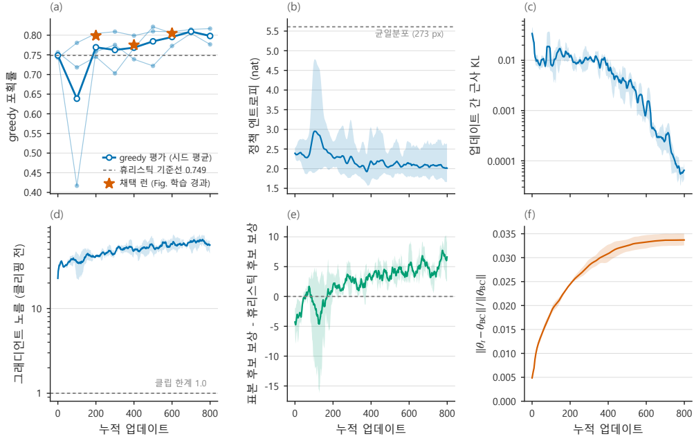
Figure 15: 수렴 진단 — 채택 런과 같은 설정을 시드 3개로 다시 돌린 학습 동역학. 굵은 선은 시드 평균, 띠는 시드 간 최소 최대, 시계열은 20 업데이트 이동평균이다. (a) 100 업데이트 마다의 greedy 포획률(얇은 선은 시드별, 원은 평균, 별표는 채택 런의 평가점, 회색 파선은 같은 프로토콜로 랜 휴리스틱 기준선 0.749). (b) 1단계 픽셀 분포의 엔트로피. 파선은 유효 픽셀 중앙값 273개의 균일분포. (c) 갱신 전후 정책의 근사 KL 발산(같은 관측·같은 표본 후보, 로그축). (d) 클리핑 전 그래디언트 노름(로그축) — 항상 클립 한계 위에 있어 수렴 지표가 아니다. (e) 표본 후보 보상에서 휴리스틱 후보 보상을 뺀 값. 0 을 넘으면 정책의 표본이 휴리스틱을 앞선다. (f) 행동복제 초기점으로부터의 상대 파라미터 이동 거리.
