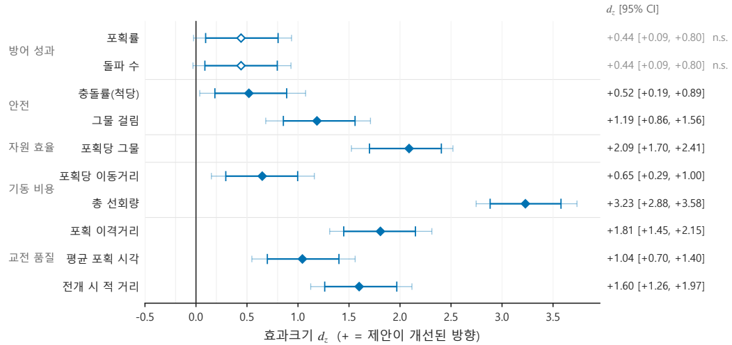
Figure 18: 제안(11m_unet@Gemini) 대 기준선(heur_heur)의 전 지표 효과크기. 마름모가 점추정이고, 굵은 선이 95% 신뢰구간, 그 바깥의 옅은 선이 지표 10개에 대한 Bonferroni 보정 구간(99.5%)이다. 속이 찬 표식은 보정 구간까지 0을 배제한 지표이며, 속이 빈 돌(포획률·돌파 수)은 보정을 건디지 못해 n.s.로 적었다 — Table 8의 단검 표시와 같은 판정이다. 부호는 개선 방향이 항상 양수가 되도록 통일하였다(낮을수록 좋은 지표는 뒤집었다). d_z 의 구간은 평균차의 BCa 신뢰구간을 sd(d) 로 나눈 것이므로, 이 그림이 0을 배제하는 것과 Table 8의 평균차 구간이 0을 배제하는 것은 같은 사건이다. 포획률의 효과크기가 10개 지표 중 최하위권이라는 점이 이 그림의 요지이다.
