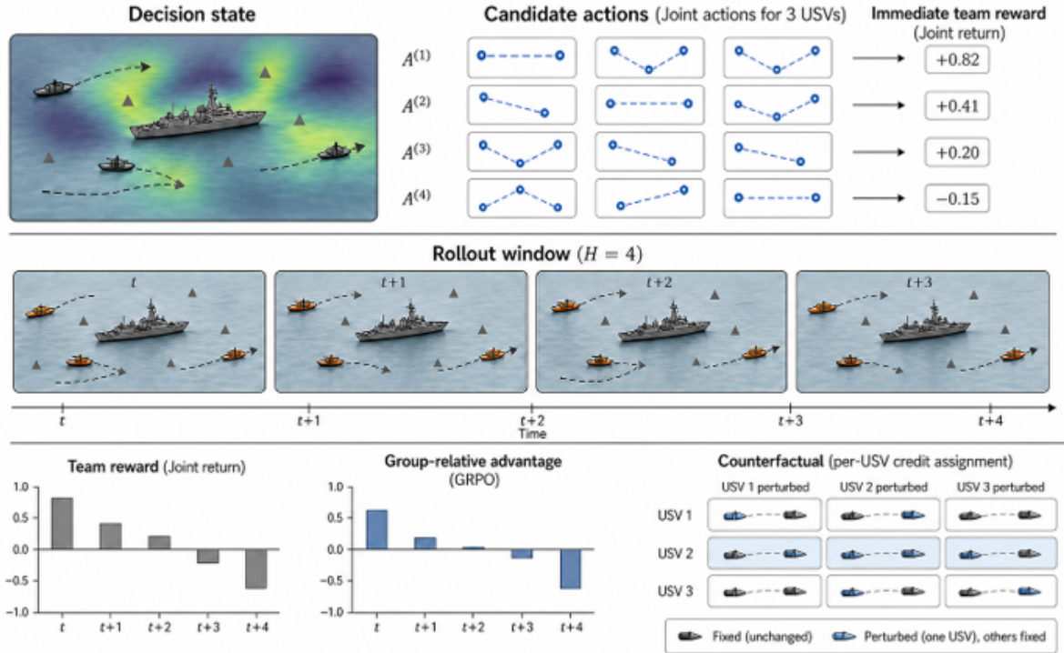
Figure 11: 가치망 없는 다중 방어정 그룹 상대 최적화의 한 갱신. 위: 한 결정 상태에서 G 개의 결합 행동 후보를 표집하고, 각 후보를 시뮬레이터에서 공통 구간만큼 실제로 진행시켜 팀 보상을 얻는다. 가운데: 후보 평가에 쓰이는 롤아웃 창. 아래 왼쪽·가운데: 팀 보상을 후보 간 상대 비교로 이득으로 바꾼다 (식 (9)). 아래 오른쪽: 반사실적 크레딧 — 한 척의 행동만 바꾸고 나머지는 고정한 채 시뮬레이터를 다시 진행시켜, 그 차이를 그 배의 몫으로 돌린다 (§4.4). 그림은 기전 전달을 위해 후보 수와 창을 G = 4 , H = 4 로 줄여 그렸으며 실제 학습은 G = 8 , 평가 구간 180 step이다.
