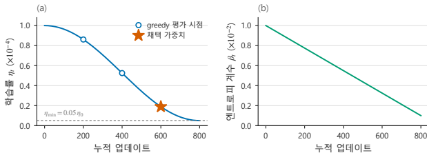
Figure 16: 학습 코드가 실제로 쓴 스케줄. (a) 식 (12)의 단일 주기 코사인 학습률. 밑 표식은 200 업데이트마다의 greedy 평가 시점, 별표는 채택 가중치(600 업데이트, \eta_t \approx 1.9 \times 10^{-5} ), 회색 파선은 \eta_{\min} 이다. (b) 엔트로피 계수 \lambda_H(t) 의 선형 감쇠 ( 0.01 \rightarrow 0.001 ).
