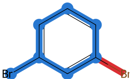
R1: 1,3-dibromobenzene
