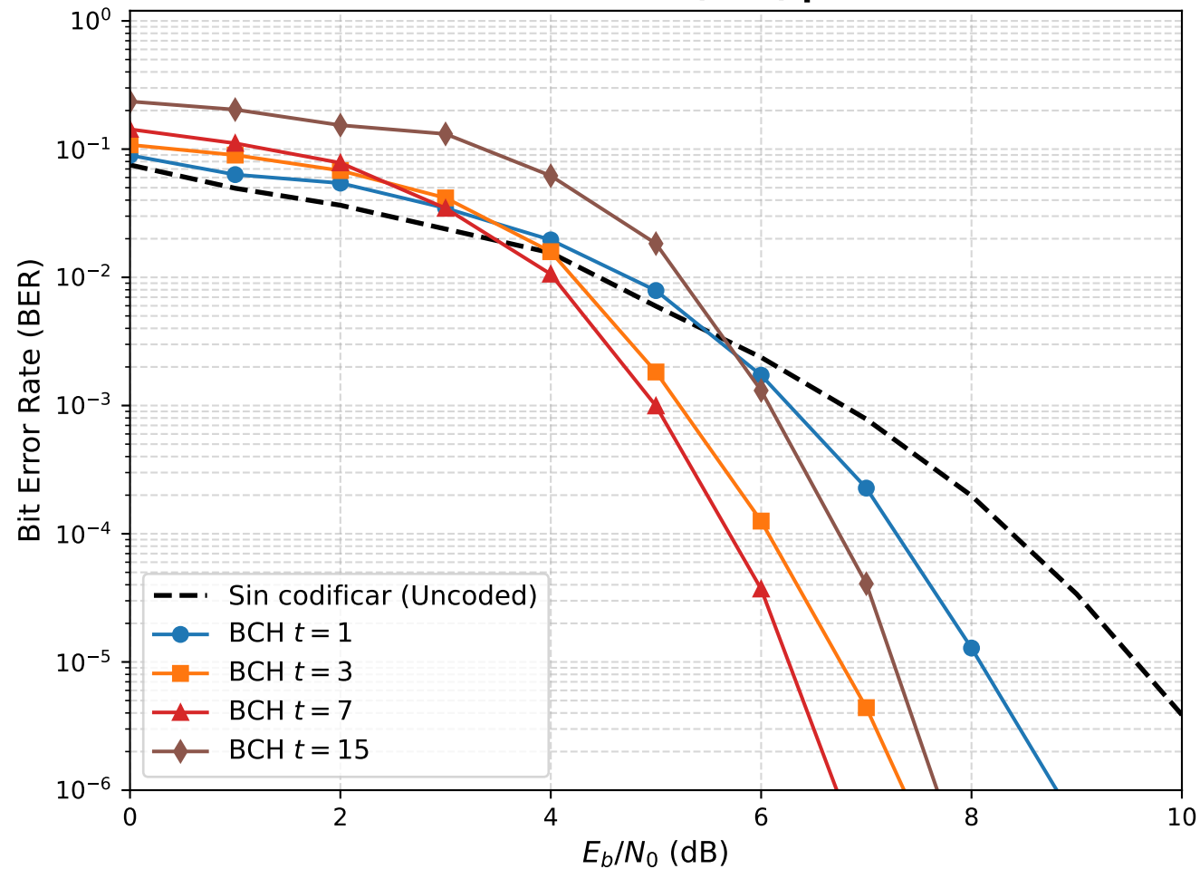
Tasa de Error de Bit (BER) para m = 7
