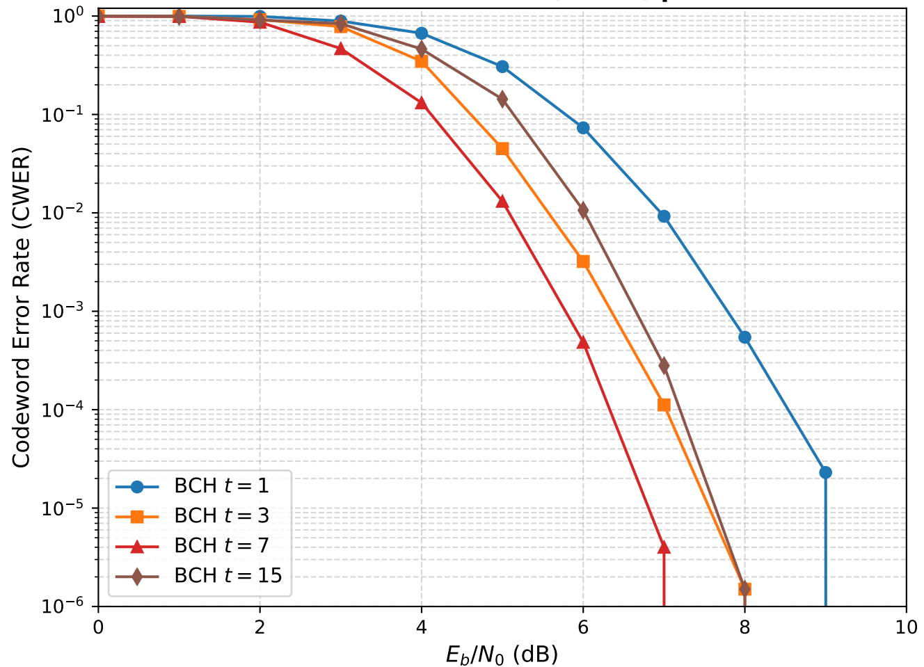
Tasa de Error de Palabra (CWER) para m = 7
