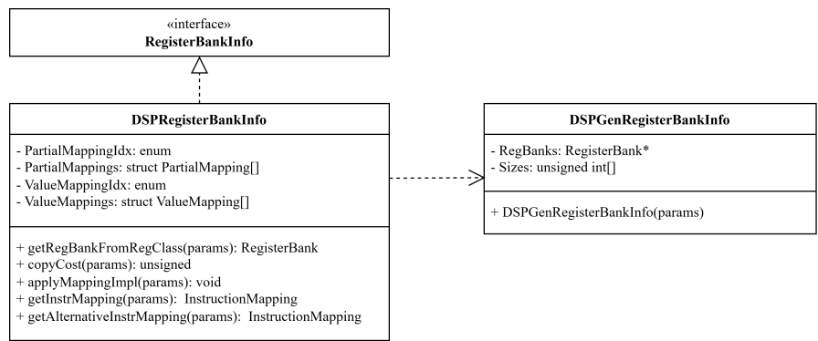
图 2-8 DSP 架构下寄存器组选择模块结构图
