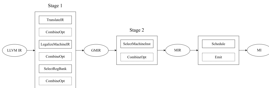
图 2-4 GlobalISel 流程图
