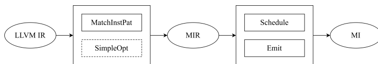
图 2-3 FastISel 流程图
