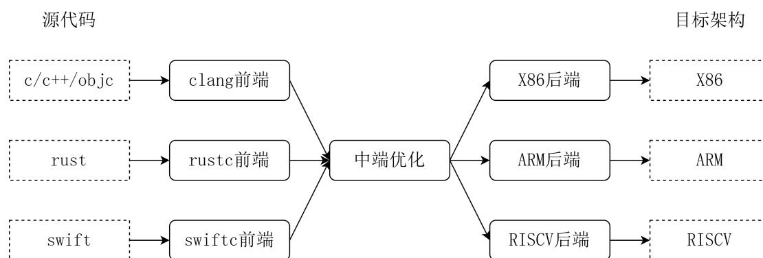
图 1-2 LLVM 架构图
