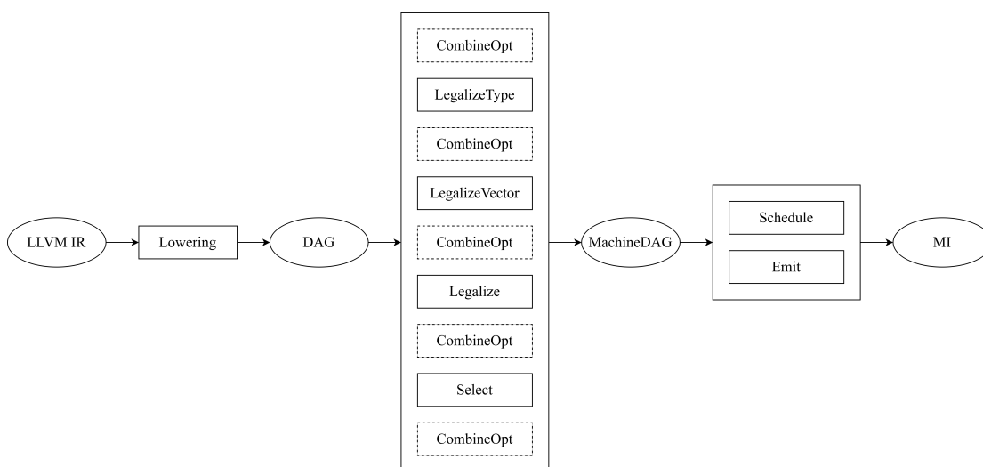
图 2-1 SelectionDAGISel 流程图
