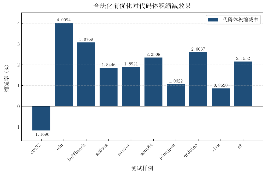
图 5-11 合法化前优化对代码体积提升效果图
