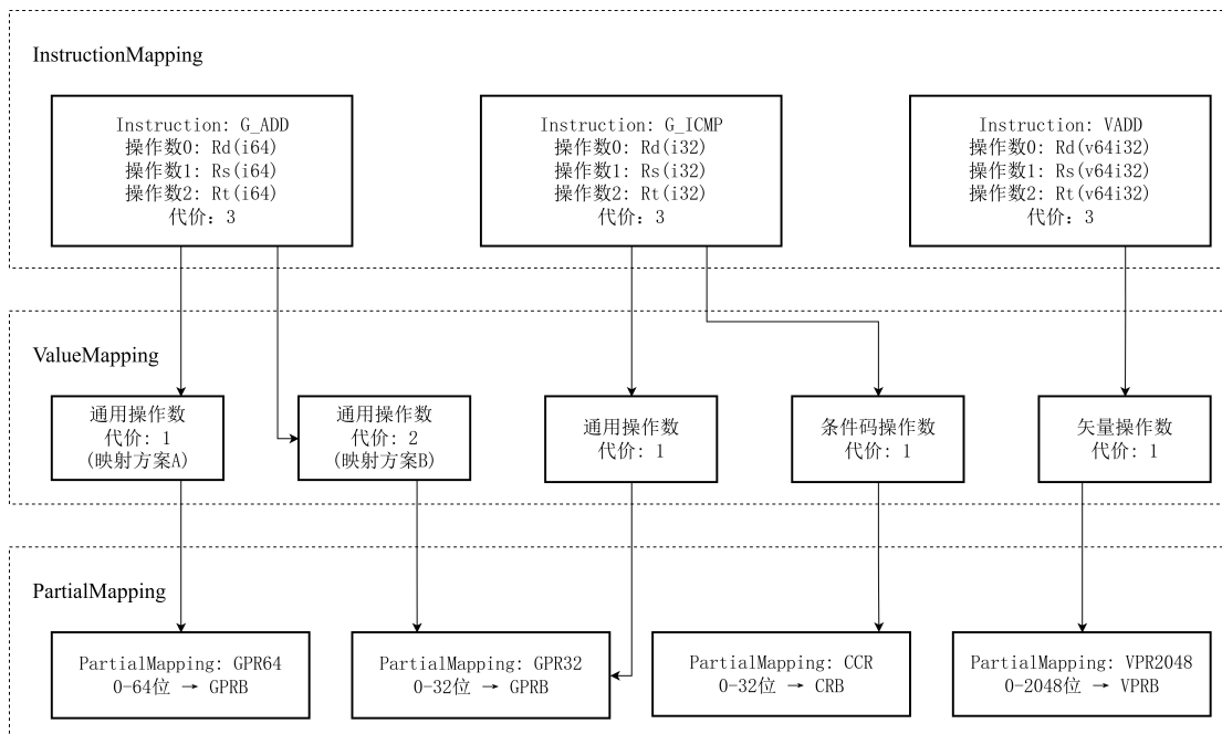
图 2-9 寄存器组分层映射结构图
