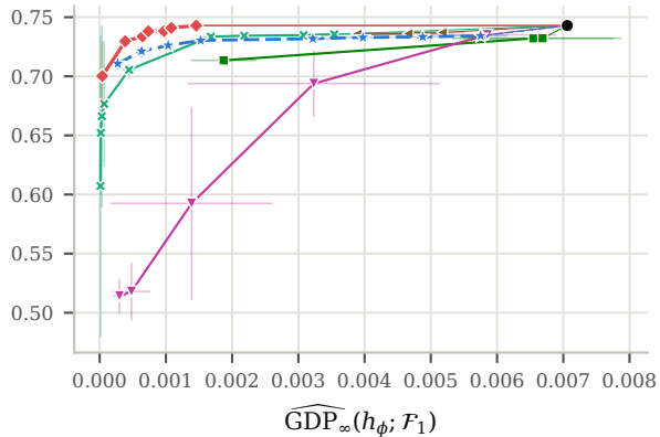
Pokec-n
