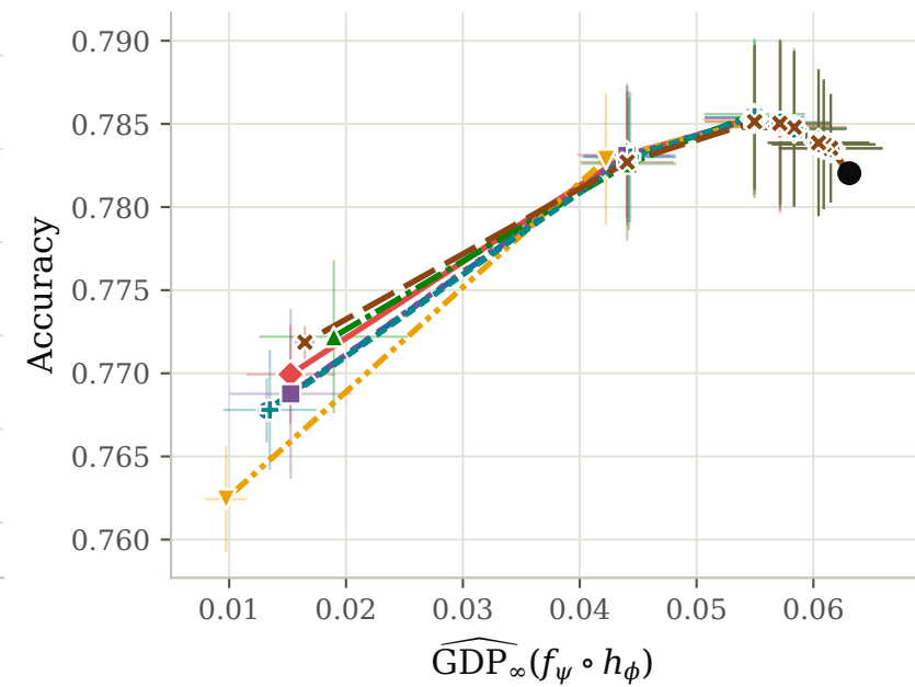
ACSIIncome
