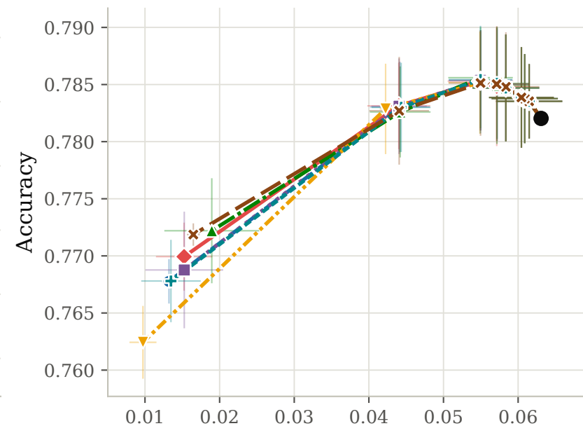
ACSIIncome
