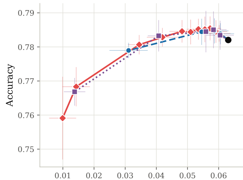
ACSIIncome
