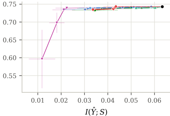
Pokec-n
