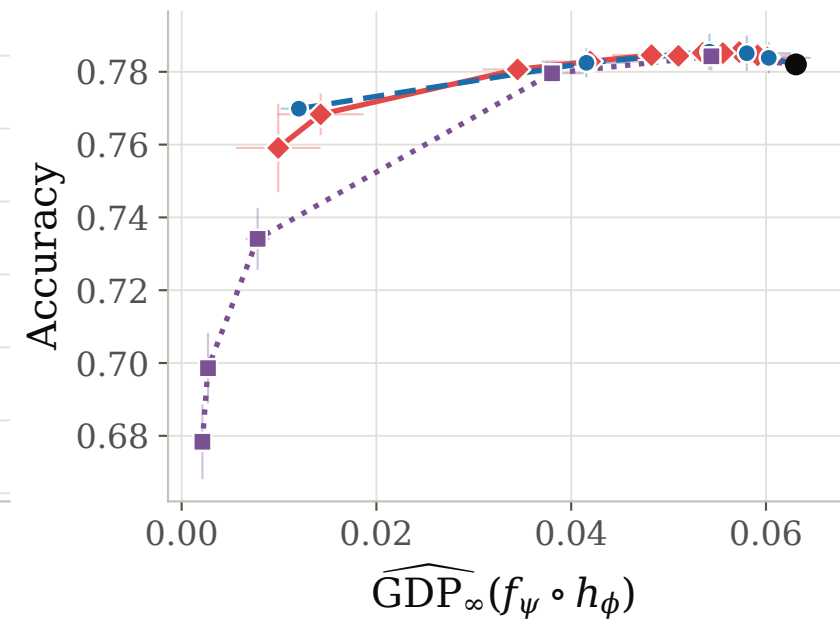
ACSIIncome
