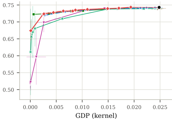
Pokec-n
