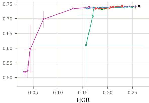
Pokec-n
