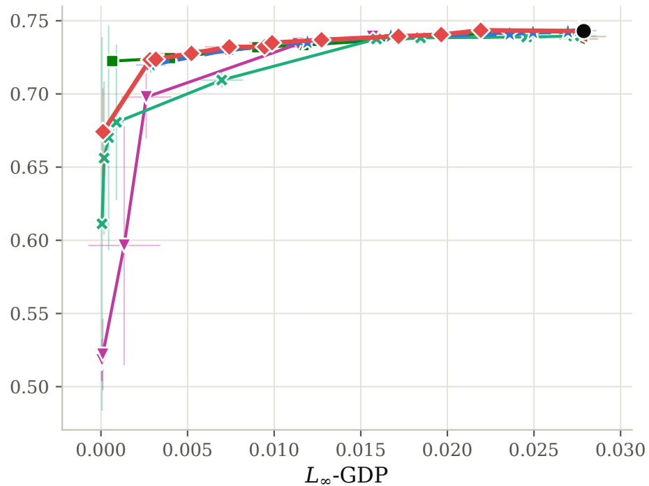
Pokec-n
