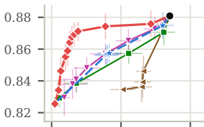
Crime (1 - MAE)
