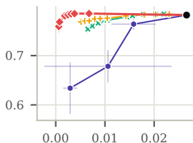
GDP_{\infty}(h_{\phi}; F_1)
