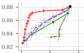
Crime (1 - MAE)
