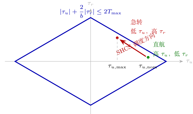
(a) 推进器可行域与工况迁移
