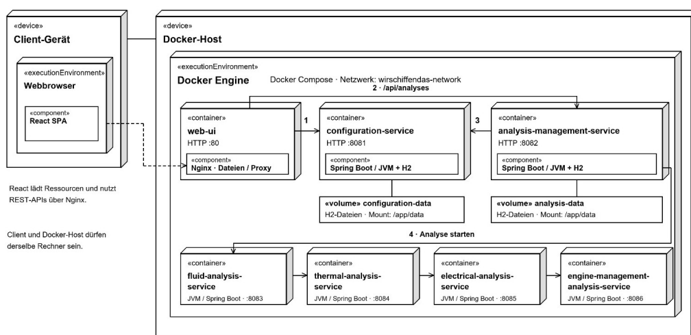
Abbildung 4: Verteilungssicht: Container, Ports und Docker-Compose-Netzwerk.
