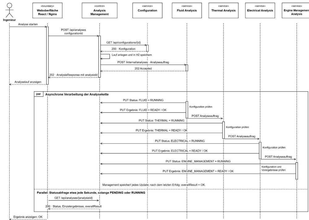
Abbildung 3: Laufzeitsicht: sequenzielle Choreographie der Analyse-Services.
