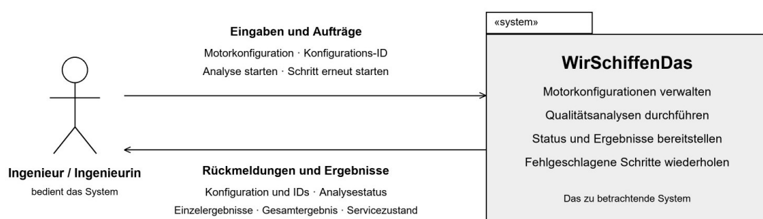
Abbildung 1: Kontextsicht: Akteur, Frontend und Engine Quality Analysis.
