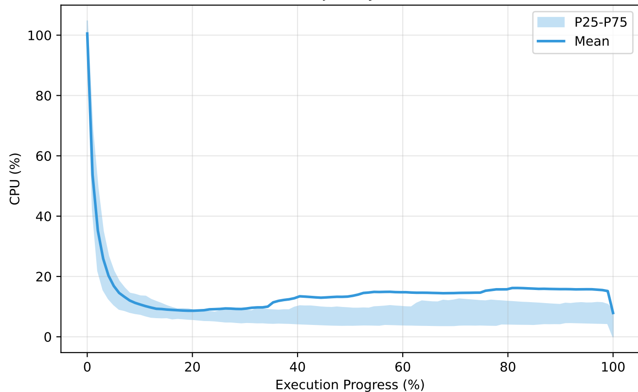
CPU Trajectory (n=33)
