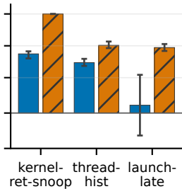
(b) RTX 5090
