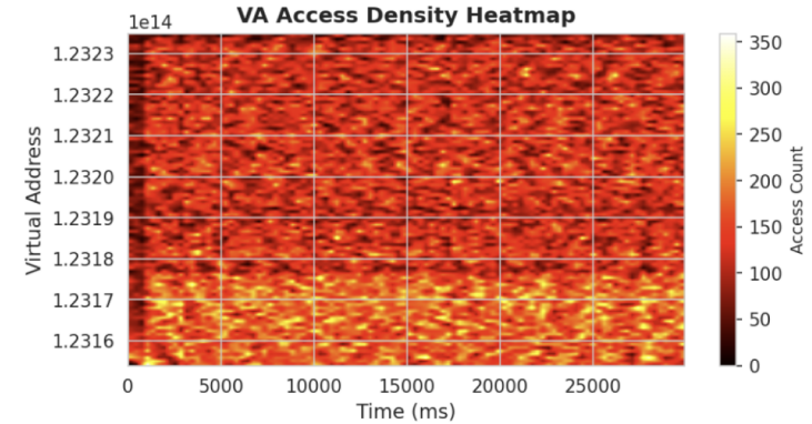
FAISS Query
