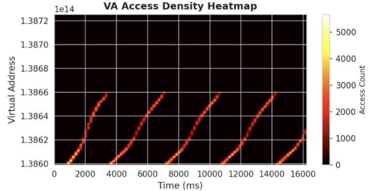
LLaMA Prefill
