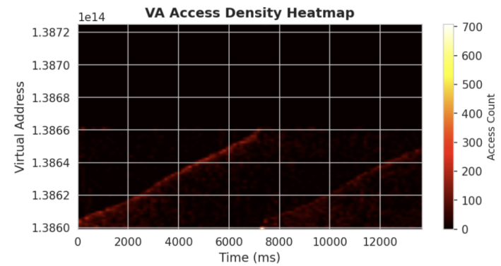
LLaMA Decode
