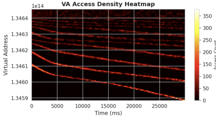
FAISS Build
