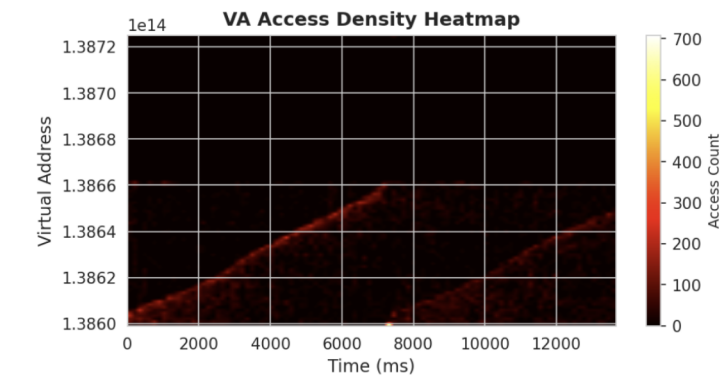
LLaMA Decode
