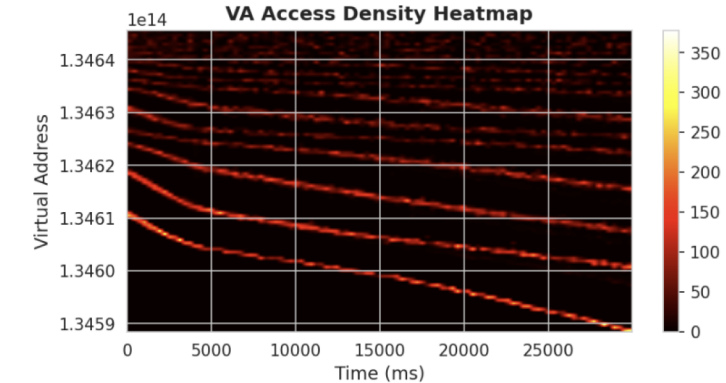
FAISS Build
