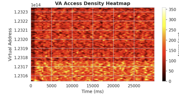
FAISS Query
