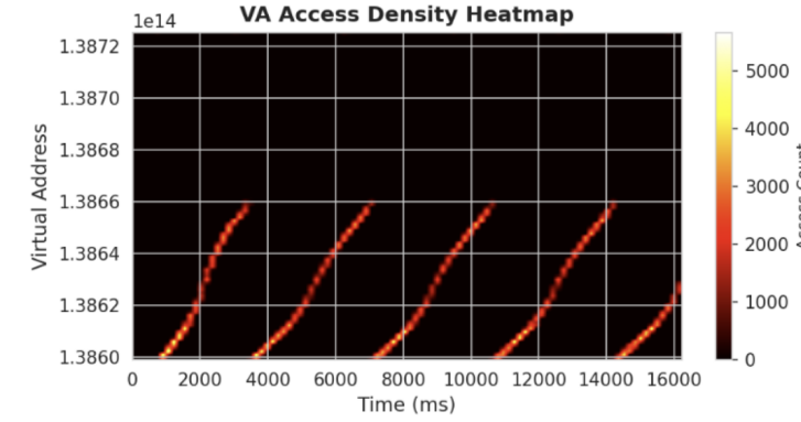
LLaMA Prefill
