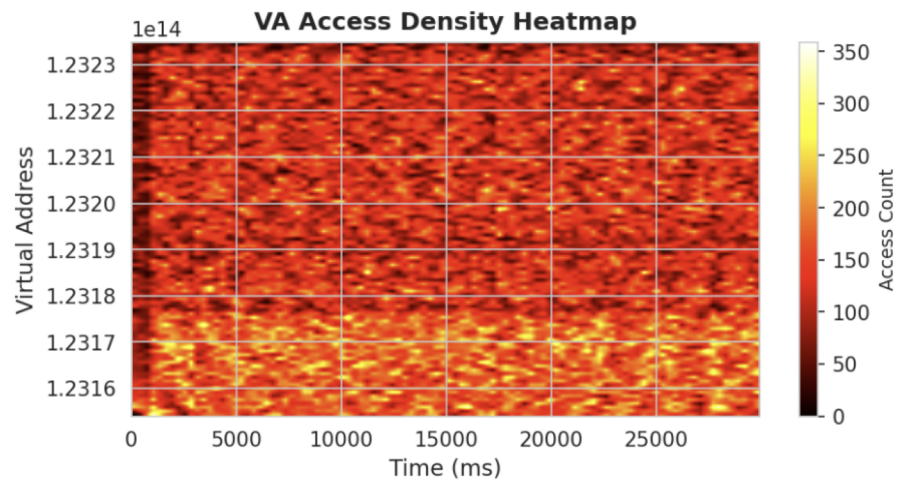
FAISS Query
