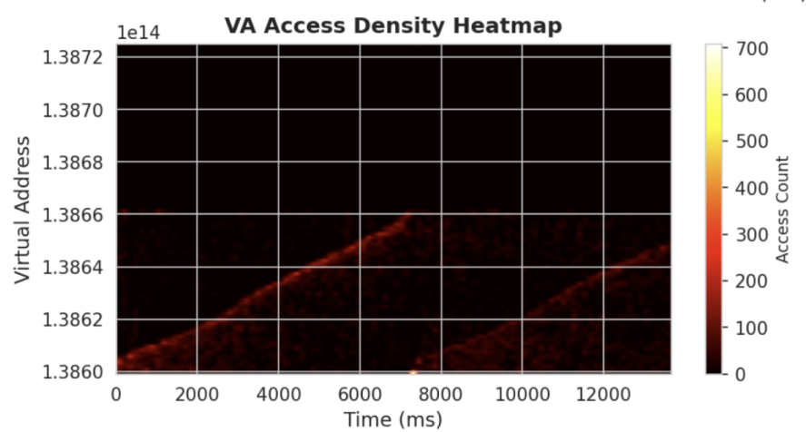
LLaMA Decode
