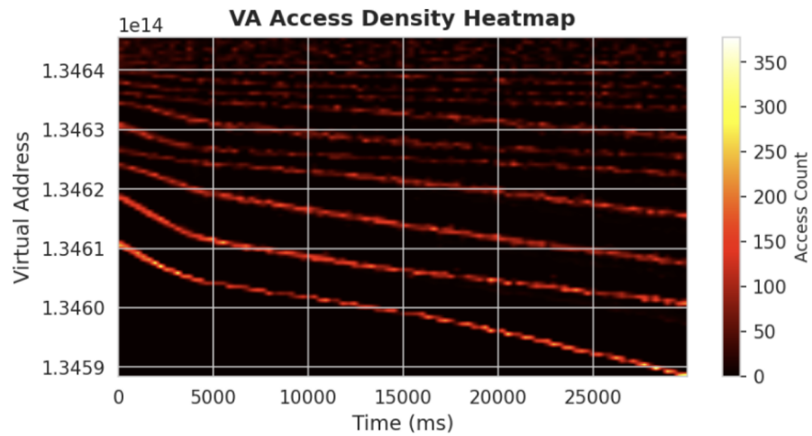
FAISS Build
