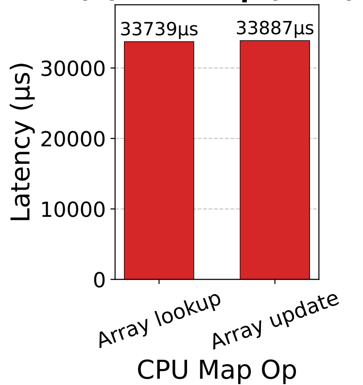
(b) CPU Map (PCIe)
