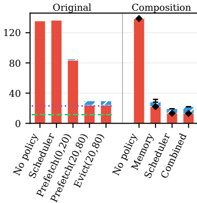
(b) GEMM
