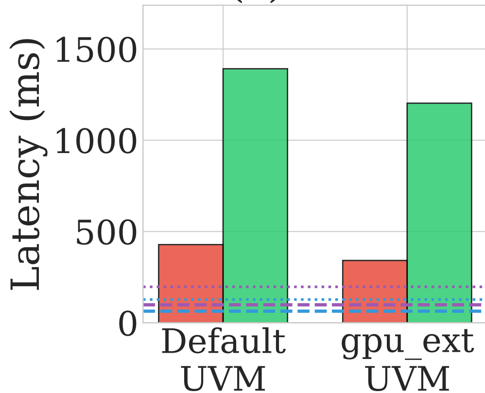
(a) TTFT
