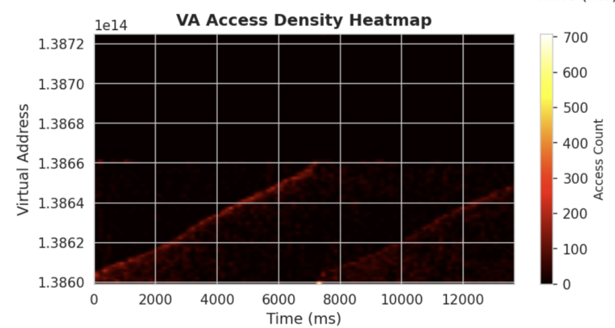
LLaMA Decode
