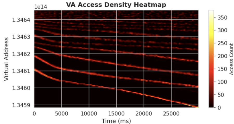
FAISS Build
