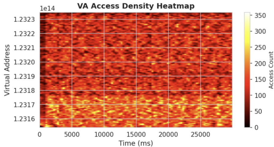
FAISS Query
