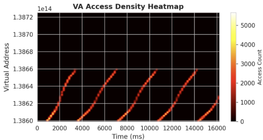
LLaMA Prefill
