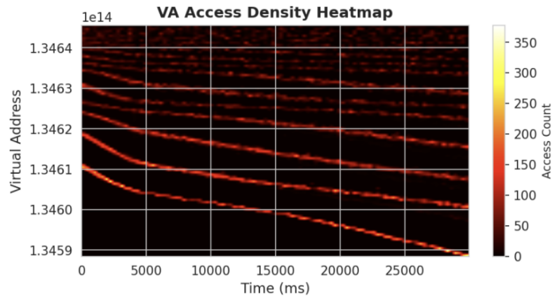
FAISS Build
