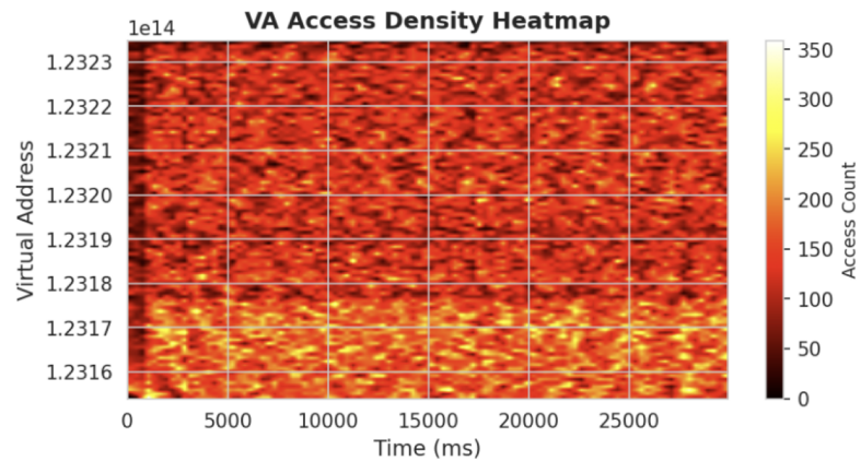
FAISS Query
