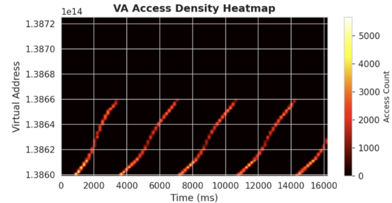
LLaMA Prefill
