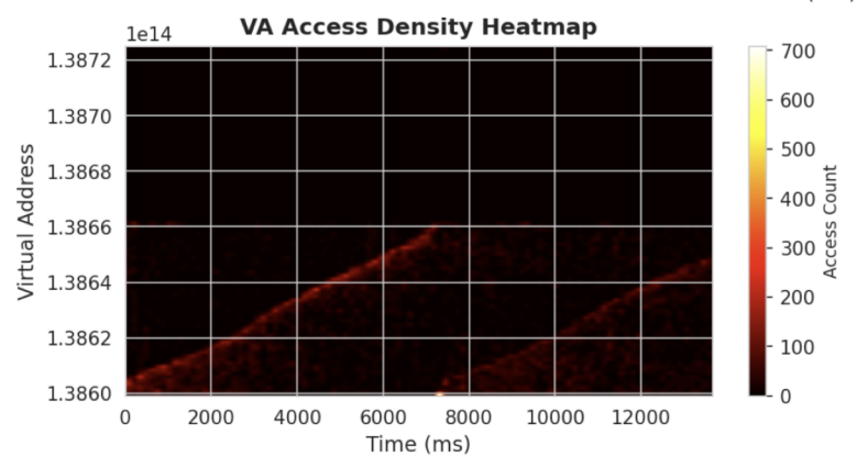
LLaMA Decode
