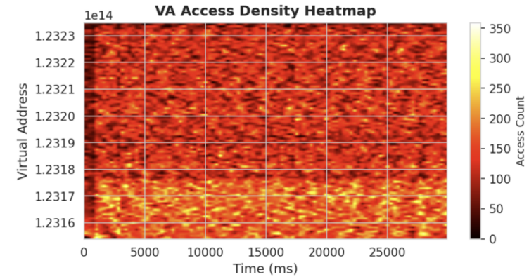
FAISS Query
