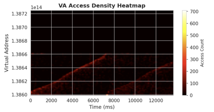
LLaMA Decode
