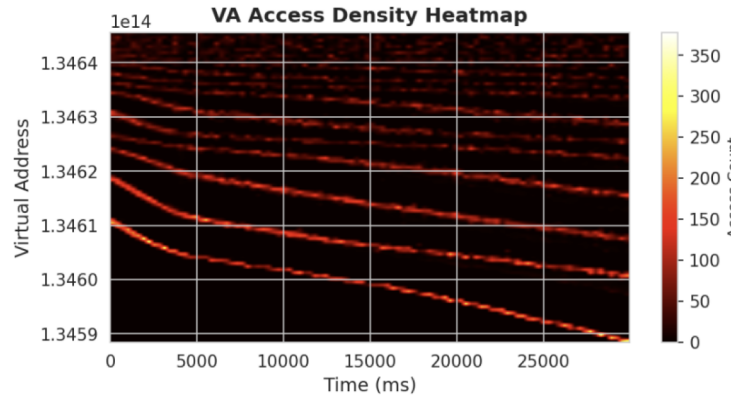
FAISS Build
