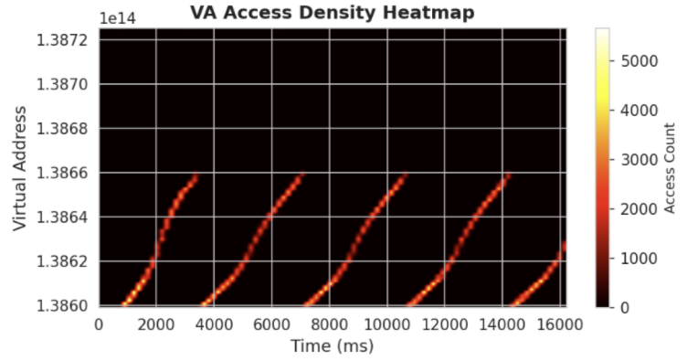
LLaMA Prefill
